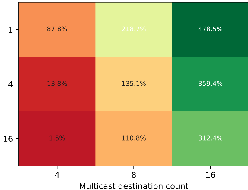
4x4 Mesh
