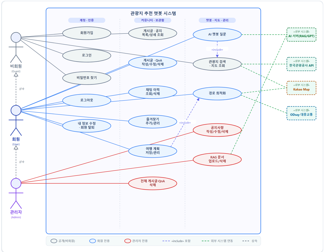
[그림 2-1] 관광지 추천 챗봇 Use-Case Diagram
