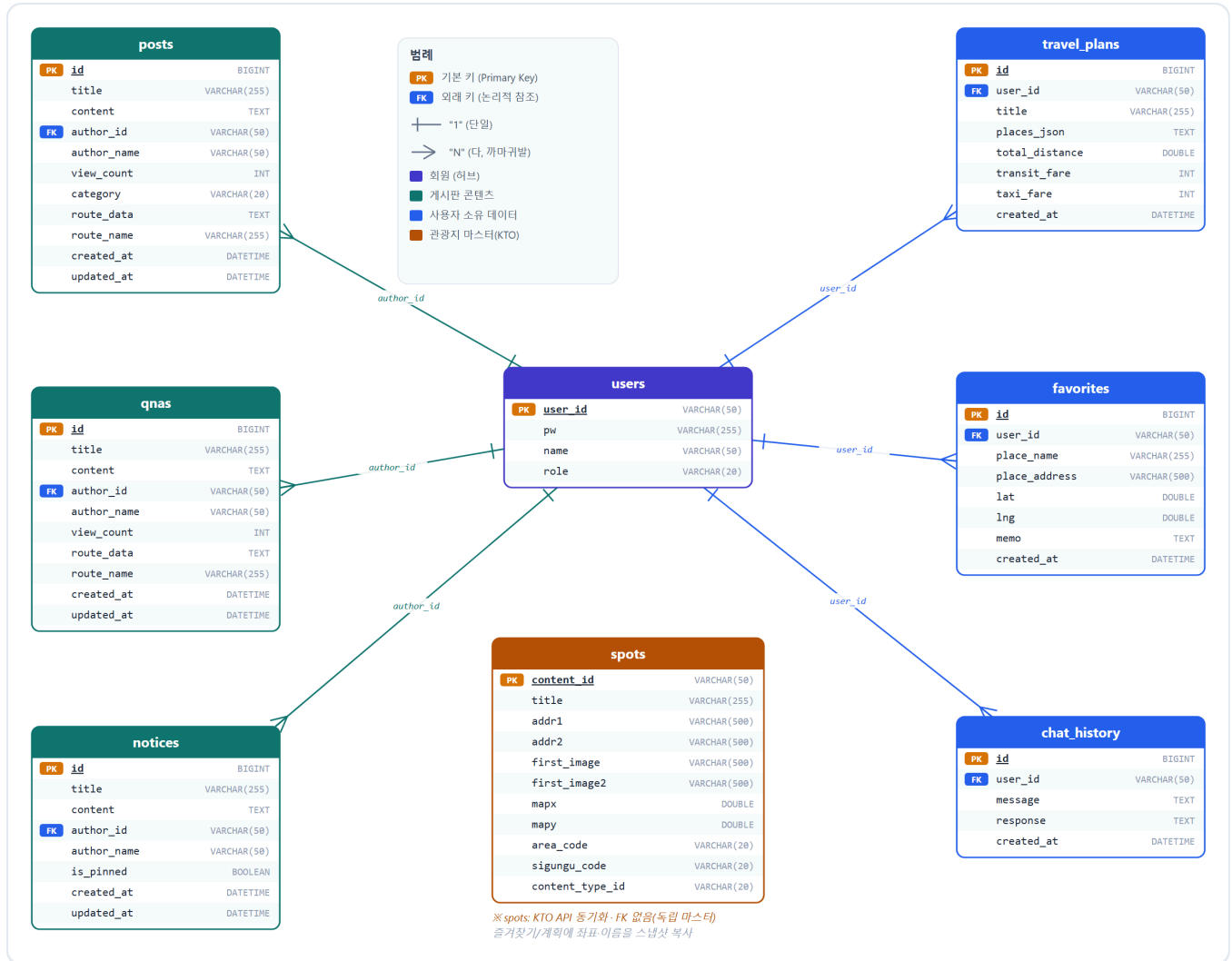
[그림 4-1] 데이터베이스 ER Diagram (Crow's Foot)
