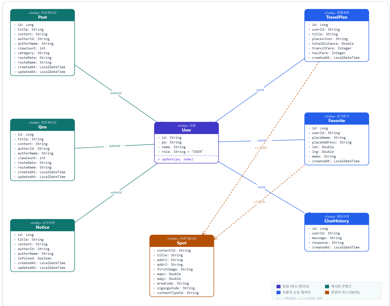
[그림 3-1] 도메인 클래스 다이어그램 (UML)
