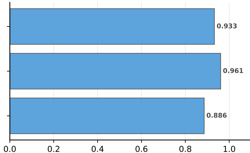
AUC
