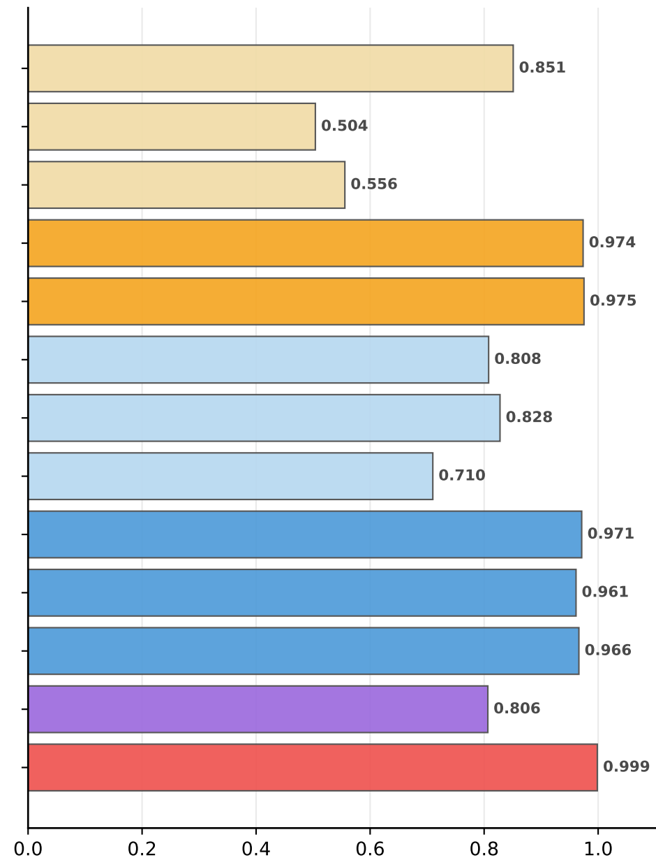
AUC
