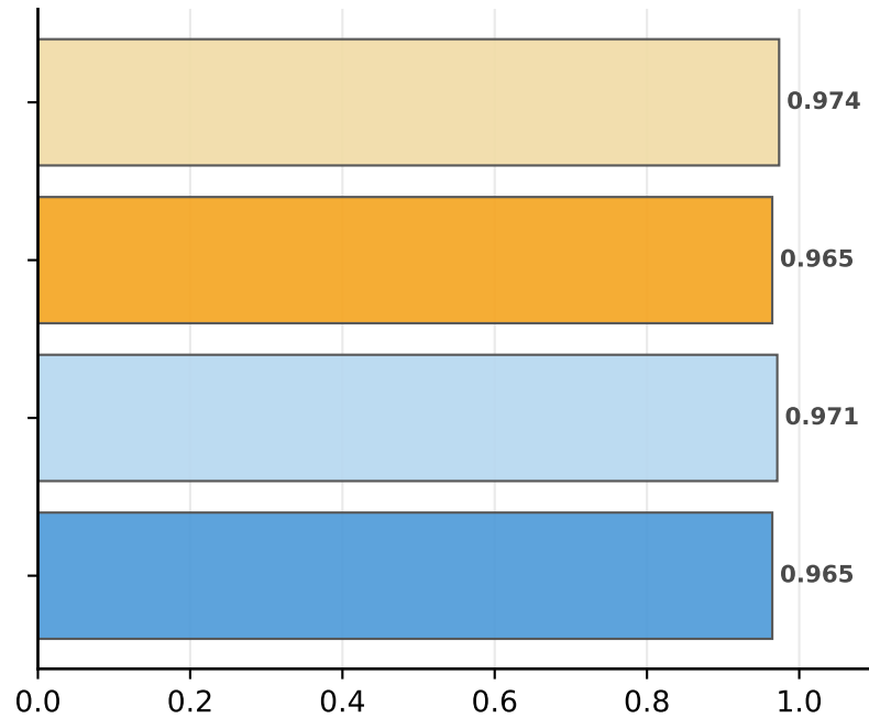
AUC
