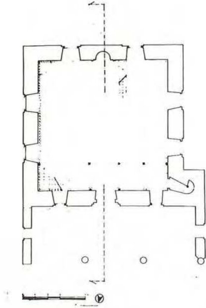
Çiz. 2 — Kurşunlu Cami, plan
