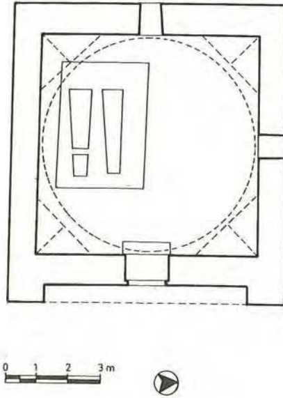
Çiz. 8 — Süleyman Şah Türbesi, plan
