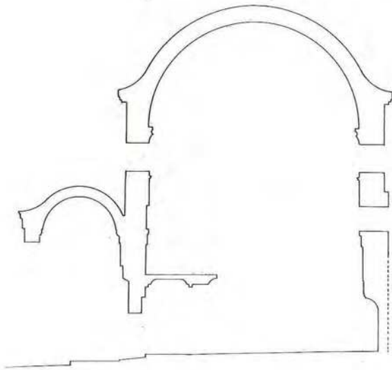
Çiz. 3 — Kurşunlu Cami, kesit
