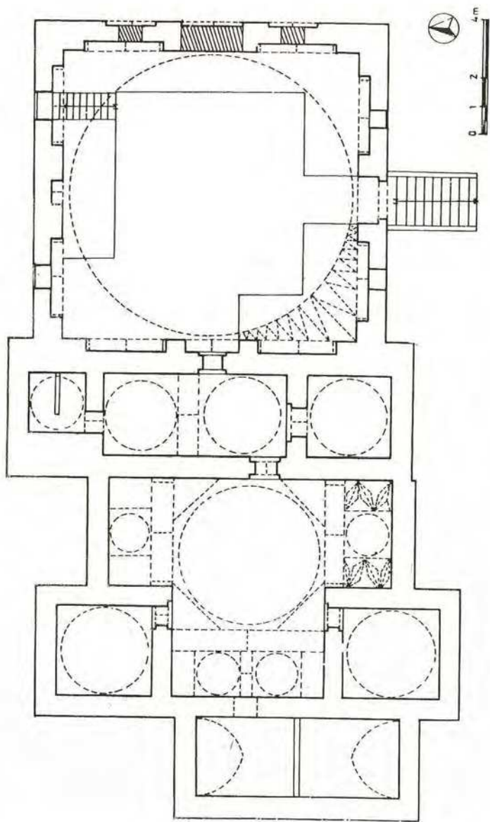
Çiz. 9 — Yeni Hamam, plan
