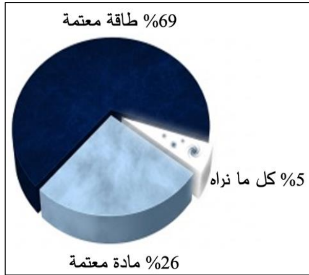
توزُّعُ المادةِ والطاقةِ في الكونِ
