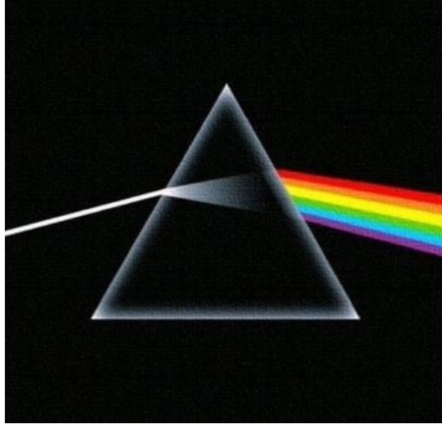
طيفُ (ألوان) الضوء المرئي
