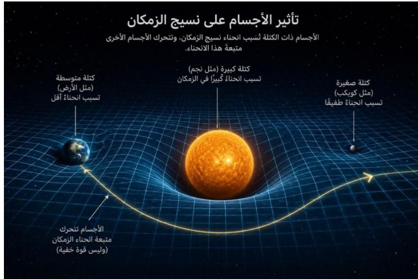
منظرٌ تصويريٌّ لتأثيرِ الأجسامِ على نسيجِ الزمكانِ
