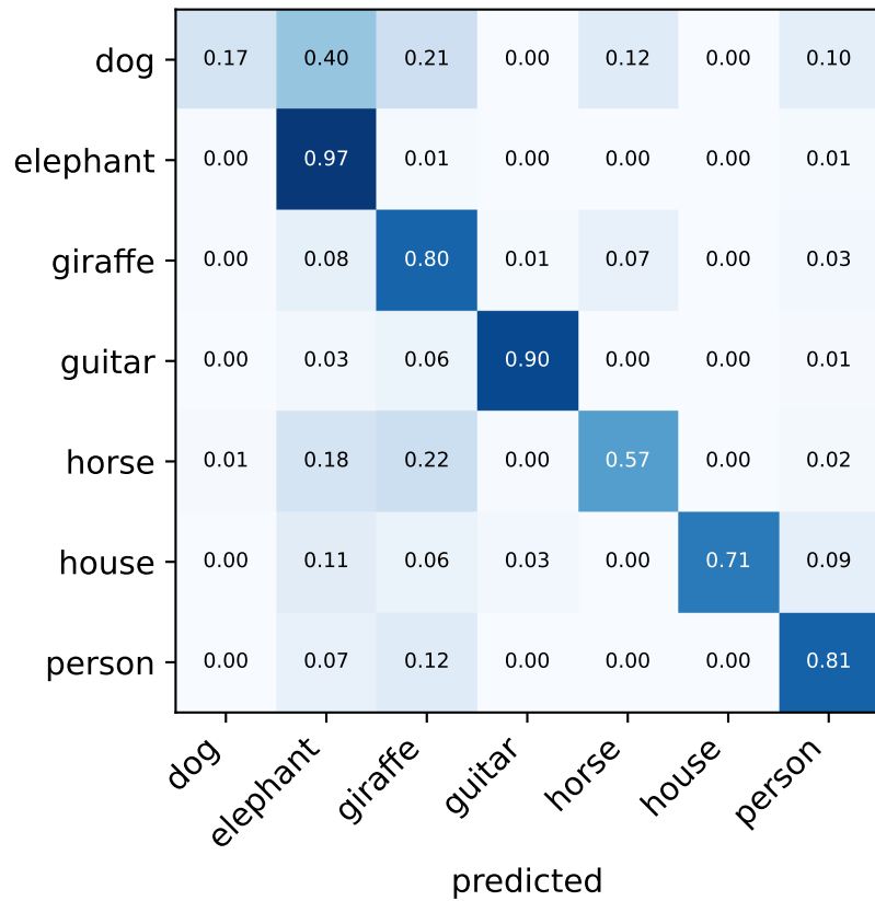
ERM (Sketch acc 0.675)
