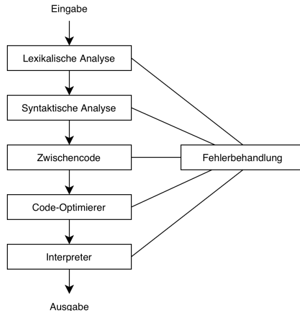
Abbildung 2.1.: Phasen eines Compilers (vereinfacht nach TODO QUELLE!)
