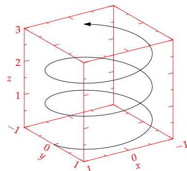
Figure 1: 这是一个边栏图。 该螺旋线由 x = \cos(2\pi z) 、 y = \sin(2\pi z) 和 z = [0, 2.7] 定义。 该图使用 Asymptote 绘制， 见 http://asymptote.sf.net/ 。
