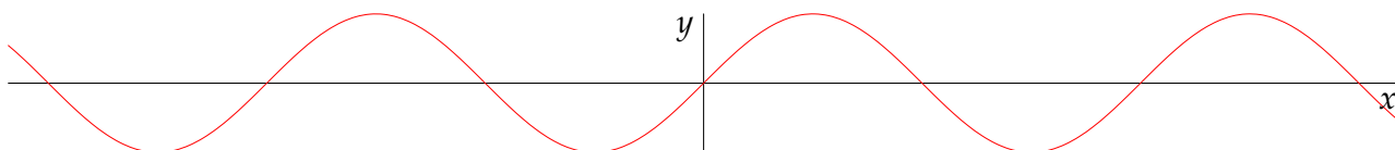
Figure 2: 这幅图展示了 y = \sin x 在大约 x = [-10, 10] 区间上的图像。请注意，这幅图占据了整页宽度。
