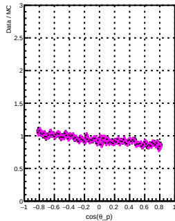
\cos\theta_p : 0.2 < \theta_e < 0.3
