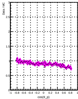
\cos\theta_p : \theta_e < 0.2
