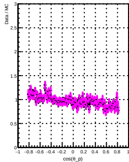
\cos\theta_p : 0.3 < \theta_e < 0.4
