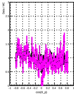
\cos\theta_p : 0.4 < \theta_e
