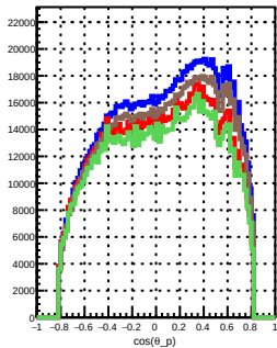
\cos\theta_p : \theta_e < 0.2
