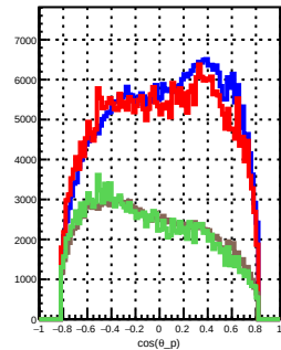
\cos\theta_p : 0.3 < \theta_e < 0.4
