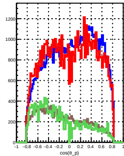
\cos\theta_p : 0.4 < \theta_e
