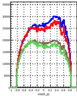
\cos\theta_p : 0.2 < \theta_e < 0.3
