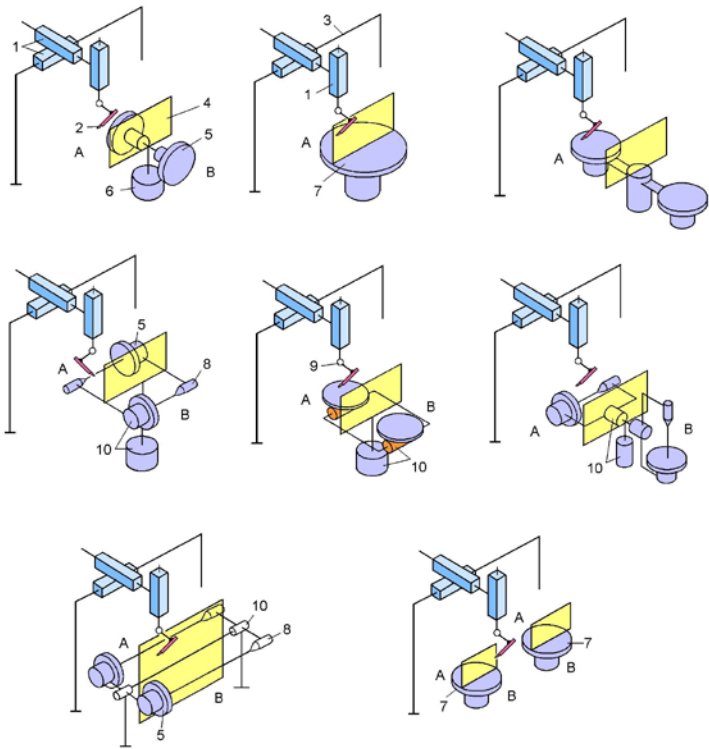
Bild 2.199 Gestaltungsbeispiele für die Peripherie an Portalroboter-Schweißplätzen. 1 Lineareinheit, 2 Schweißbrenner, 3 Portalbalken, 4 Blend- und Spritzschutzwand, 5 Drehscheibenmodul, 6 180°-Schwenkantrieb, 7 Drehtischmodul, 8 Gegenhalter-spitze, 9 Handgelenk, 10 Drehantrieb, A Arbeitsbereich, B Auf-/Abspannbereich
