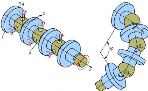
Bild 2.26 Rüsselhandgelenk. 1 Glied mit F = 3 , 2 Kreuzgelenk
