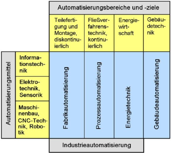
Bild 2.8 Die Fabrikautomation umfasst die Stückgut- und auch einige Anteile der Fließgutfertigung
