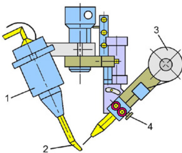
Bild 2.103 LötVorrichtung für einen Roboter und Roboterarbeitsplatz (Gesellschaft für Löttechnik). 1 LötKolbenheizung, 2 LötKolben, 3 LötDrahtrolle, 4 Drahtvorschub
