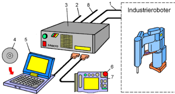
Bild 2.115 Systemkonfiguration eines Roboters ( Sankyo ). 1 Steuerleitung, 2 digitale Ein-/Ausgänge, 3 Robotersteuerung, 4 Anwendungssoftware, 5 Computer, 6 abnehmbarer Not-Aus-Taster, 7 Touch-Screen-Pendant, 8 Feldbus
