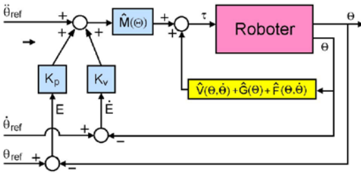
Bild 2.164 Blockbild des vorgeschlagenen nichtlinearen Regelungssystems
