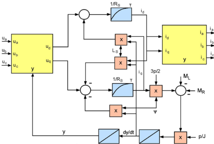
Bild 2.42 Modell einer bürstenlosen Gleichstrommaschine
