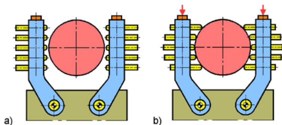
Bild 2.95 Übernahme der Werkstückform mit Abformelementen. a) Ausgangslage der Stiftfelder, b) Stifte sind auf die Werkstückform eingestellt
