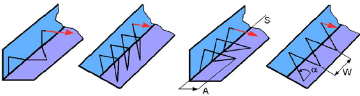
Bild 2.149 Verschiedene Pendelbewegungsmuster beim Schweißen. A Pendelamplitude, S Schweißmittelpunktsbahn, W Pendelweg, \alpha Winkel
