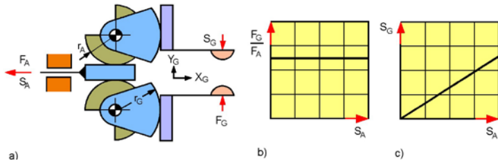
Bild 2.78 Greifkraftverlauf bei einem Parallelbackengreifer. a) kinematisches Schema, b) Greifkraftverlauf, c) Übertragungsfunktion, S_G Greifbackenweg, S_A Antriebsweg, r_A Radius des antreibenden Zahnsegmentes, r_G Radius des Greifbacken antreibenden Zahnsegmentes
