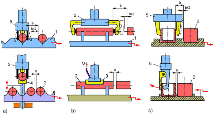
Bild 2.196 Greifbedingungen in Abhängigkeit von Greifer- und Speicherplatzausführung. a) Zusatzeinrichtung zum Ausheben, b) Anwendung eines Haftgreifers, c) Griffart verändert, 1 Flachpalette, 2 Werkstück, 3 Sauger (oder Magnet), 4 stationäres Hubprisma, 5 Klemmgreifer, a Werkstückzwischenraum, b Positionierungsfehler des Roboters, V Vakuum
