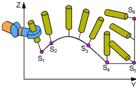
Bild 2.146 Orientierungsinterpolation. S_i Bahnstützpunkt
