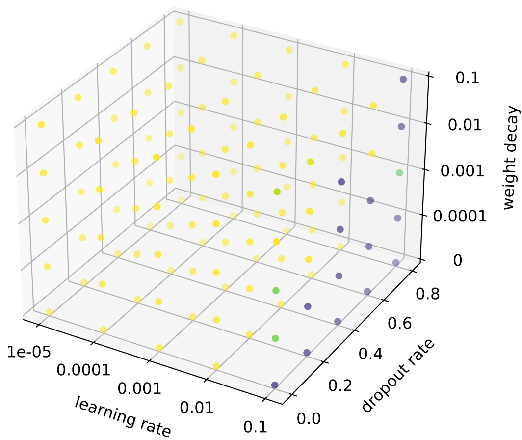
GAT
