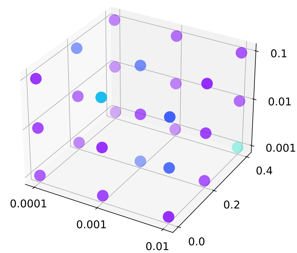
mGCN
