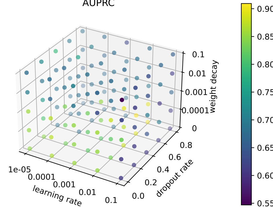
AUPRC
