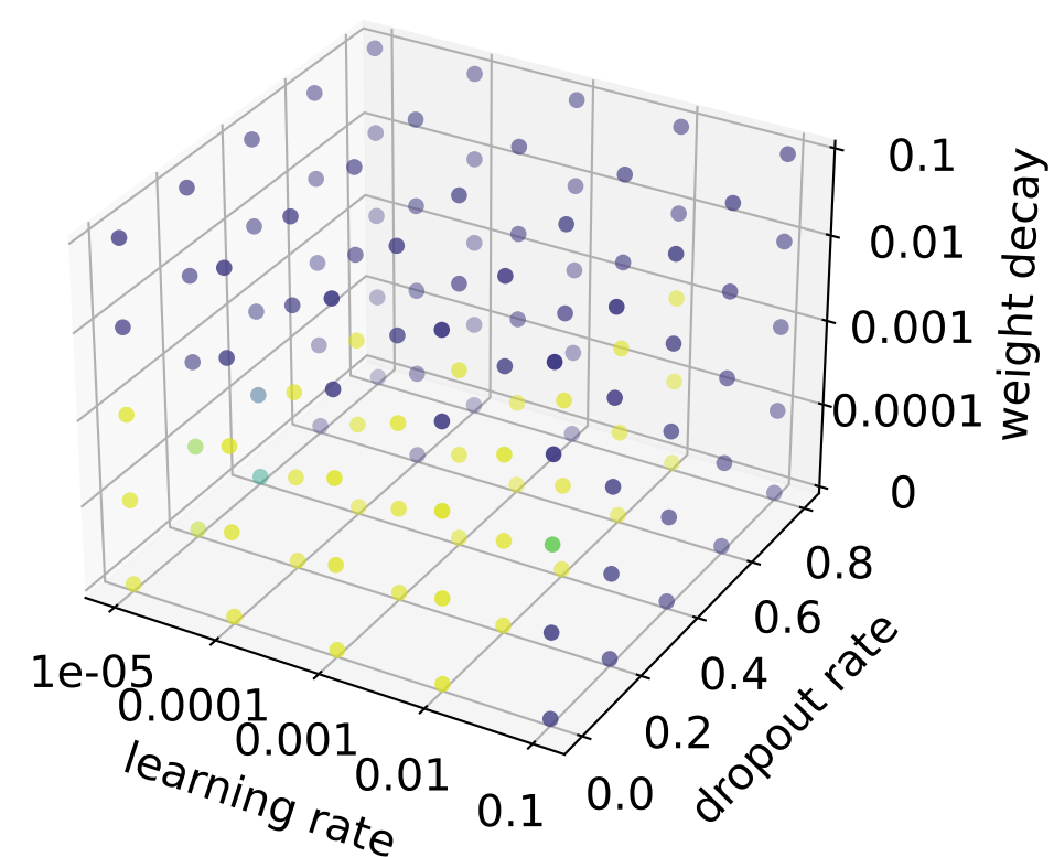
ChebNet
