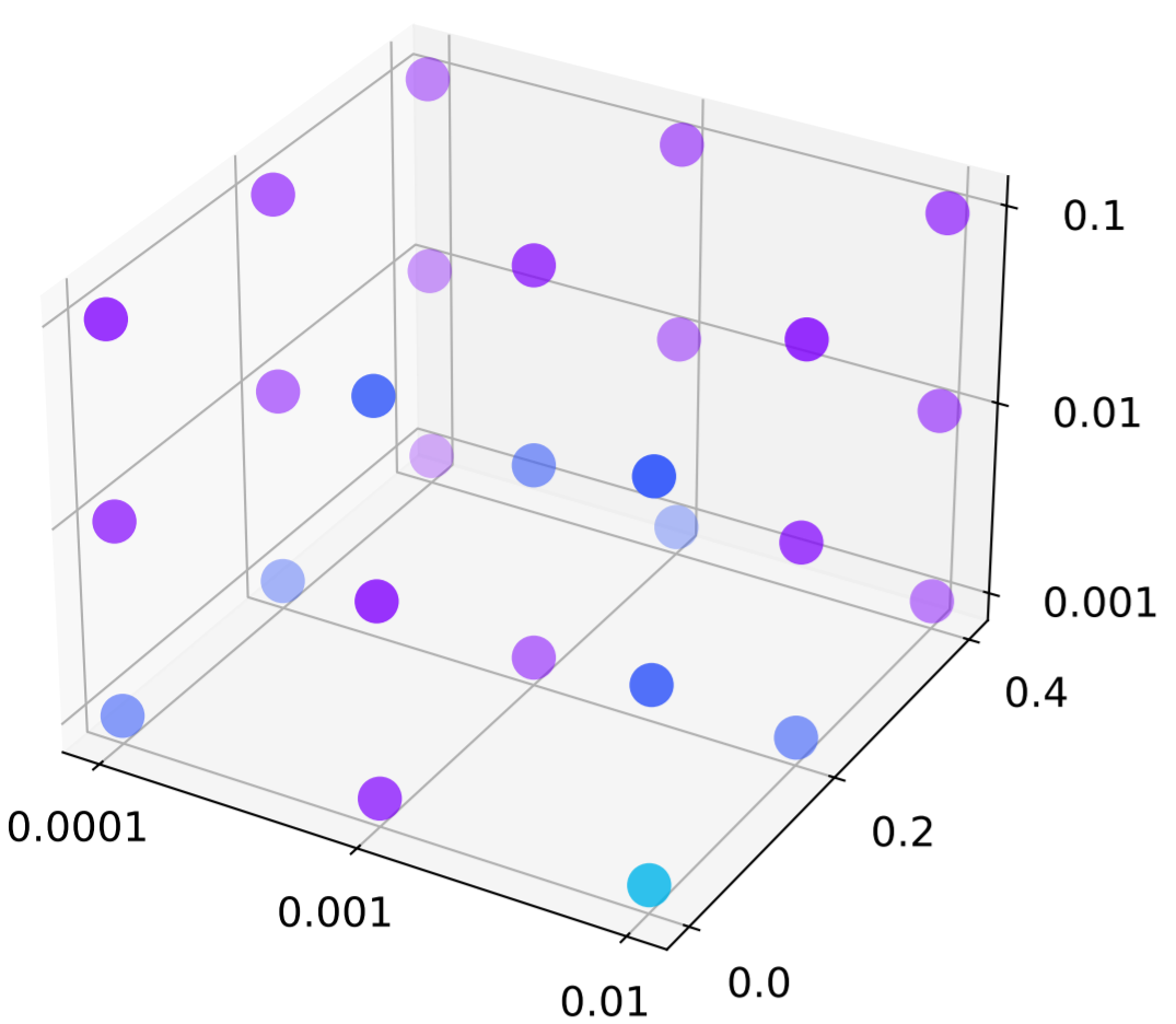
MLP
