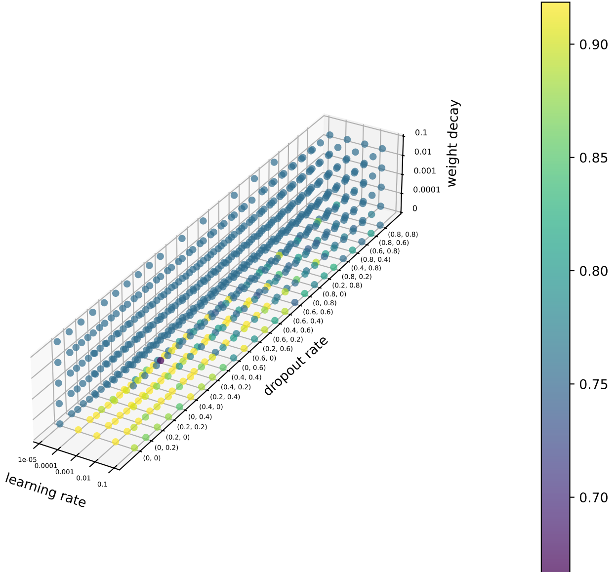
F1 scores
