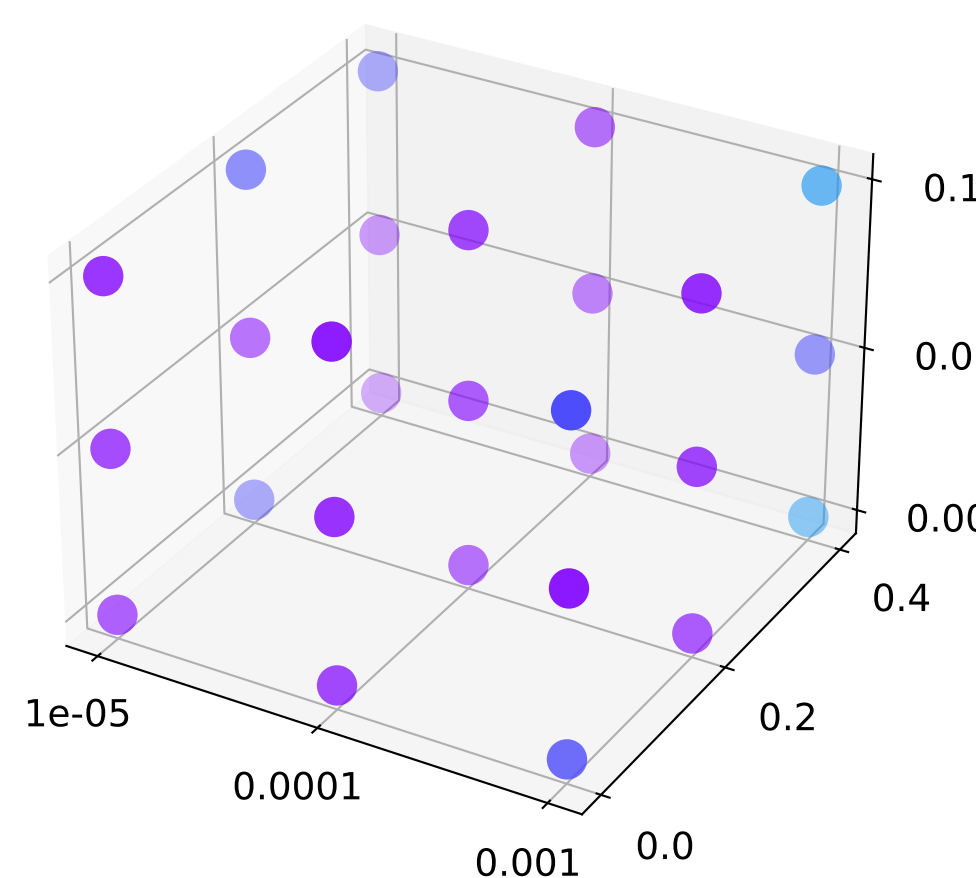
xDenseGCN
