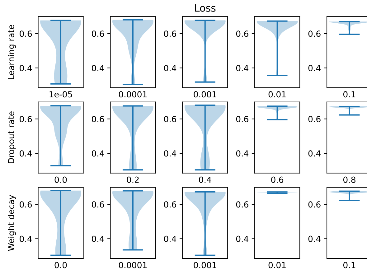
MLP (depth 32)
