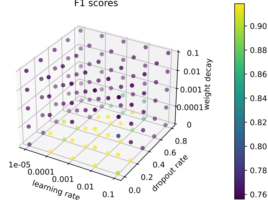
F1 scores
