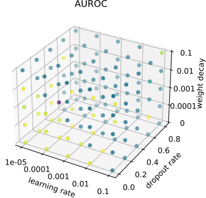
AUROC
