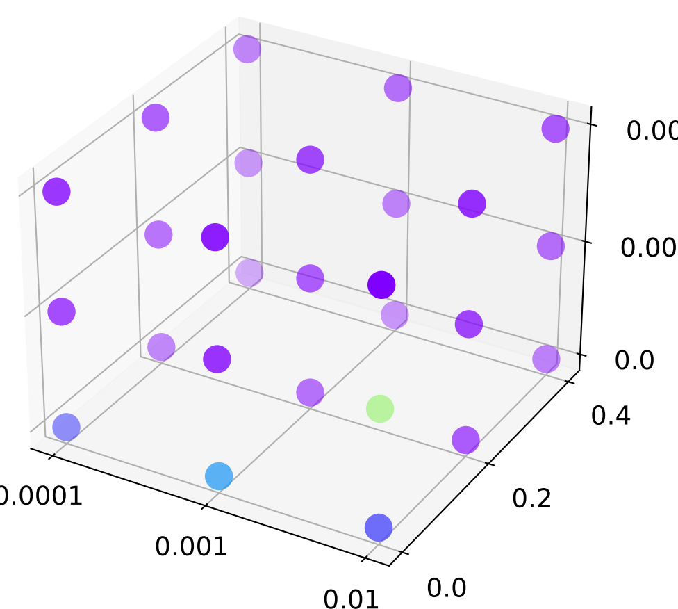
xGAT
