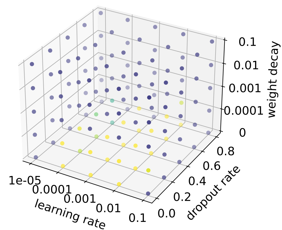
GCN
