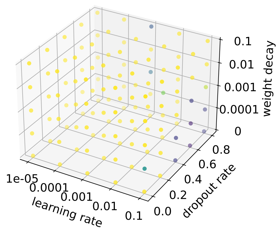
ResMLP
