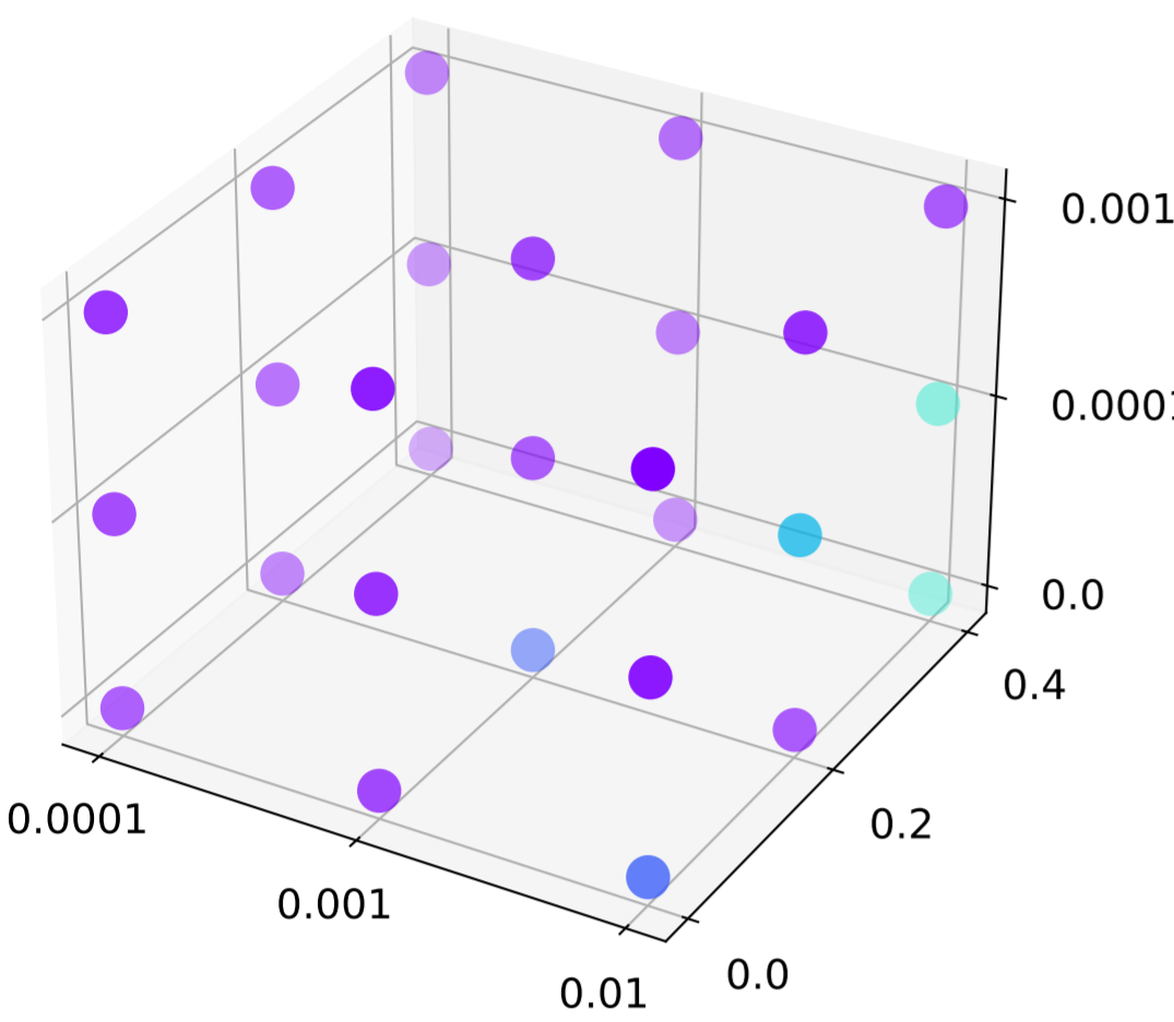
GCN
