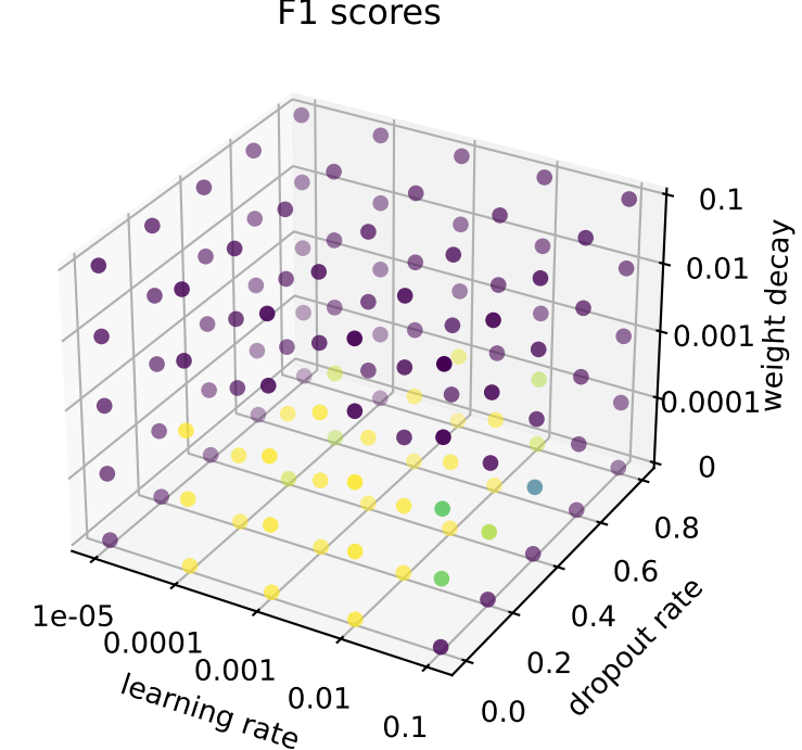
F1 scores
