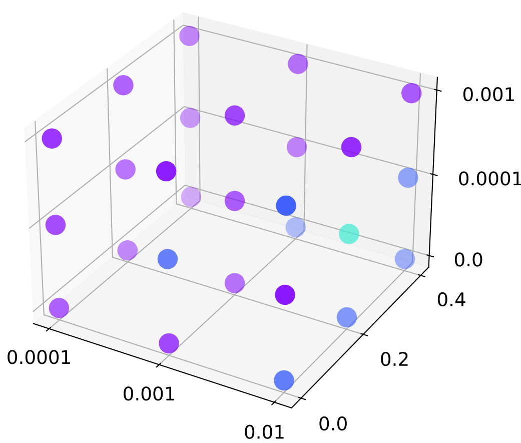
mDenseGAT
