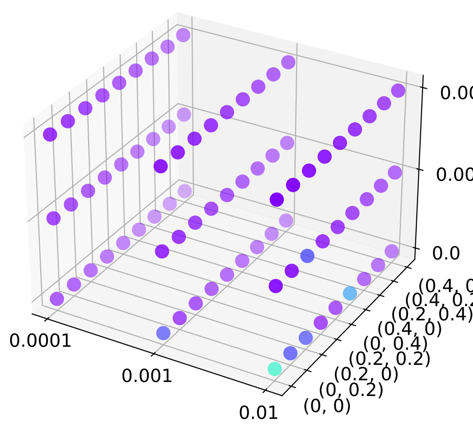
xDenseChebNet
