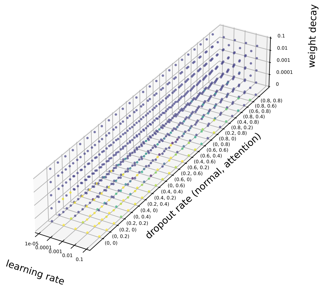
GAT
