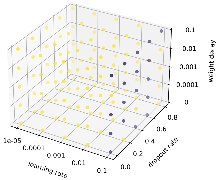
mGAT2MLP
