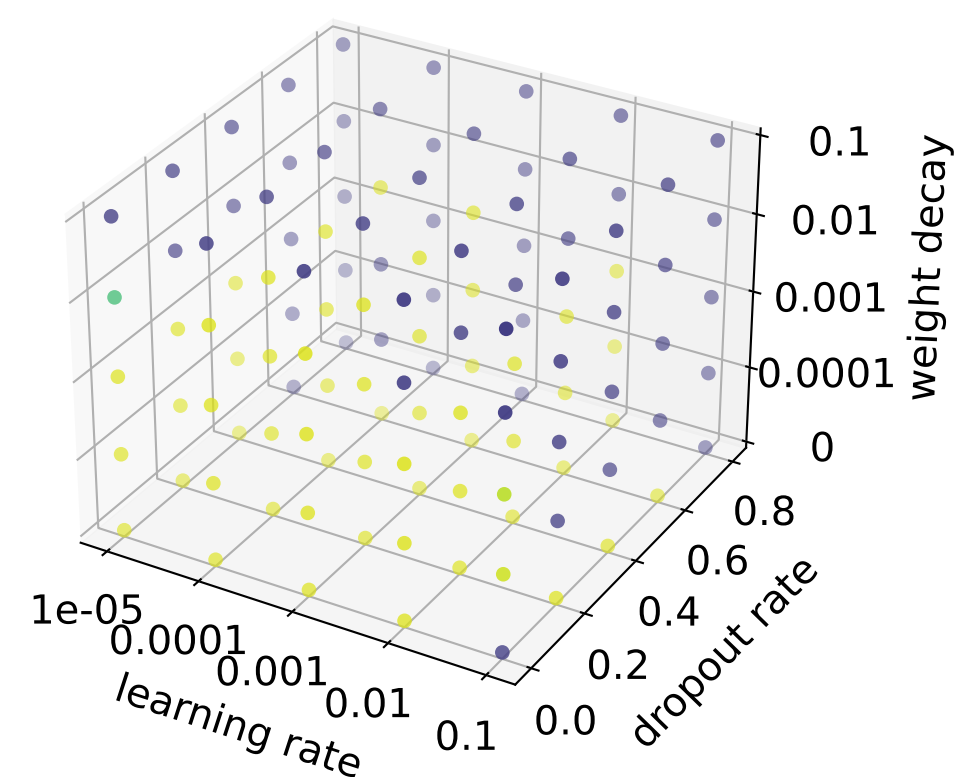
mDenseChebNet
