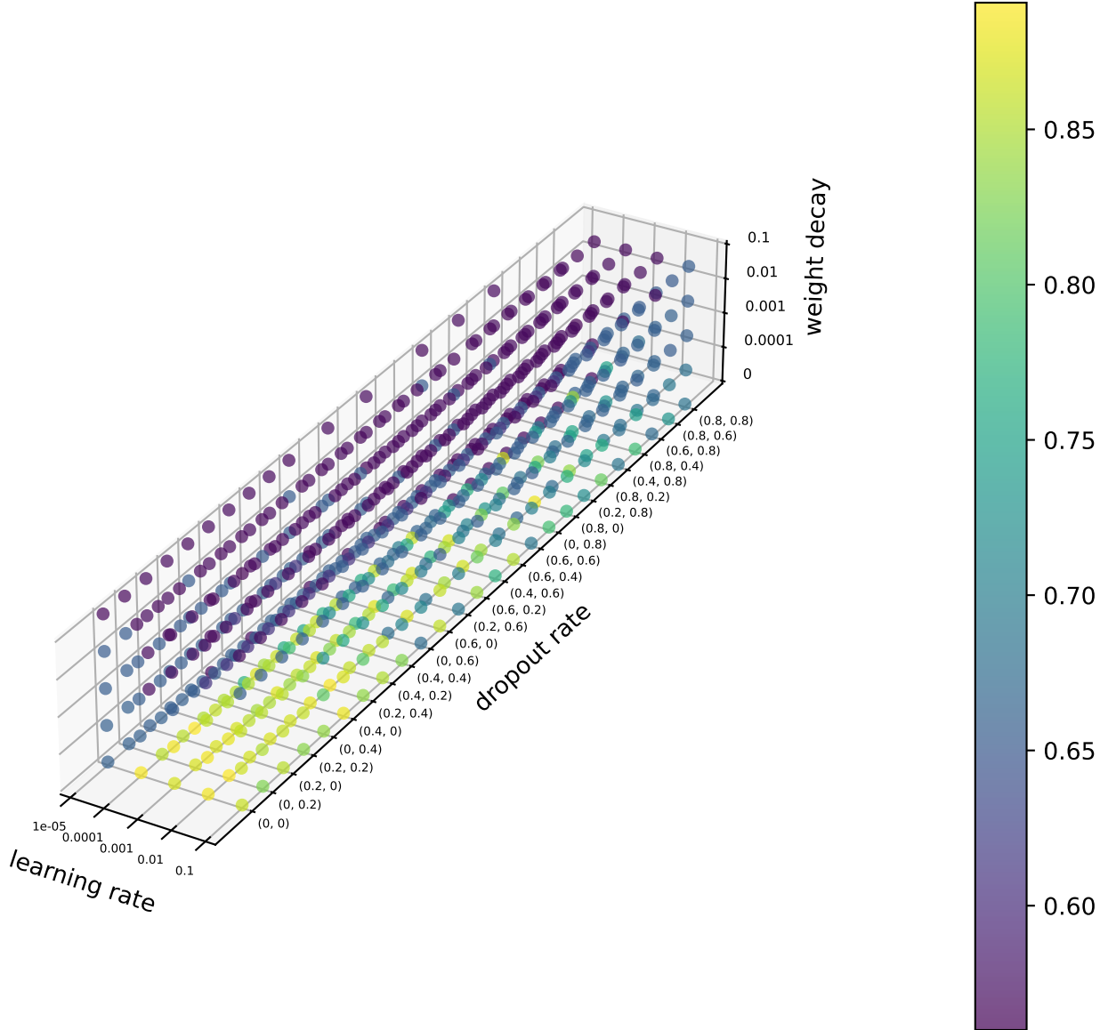
AUPRC
