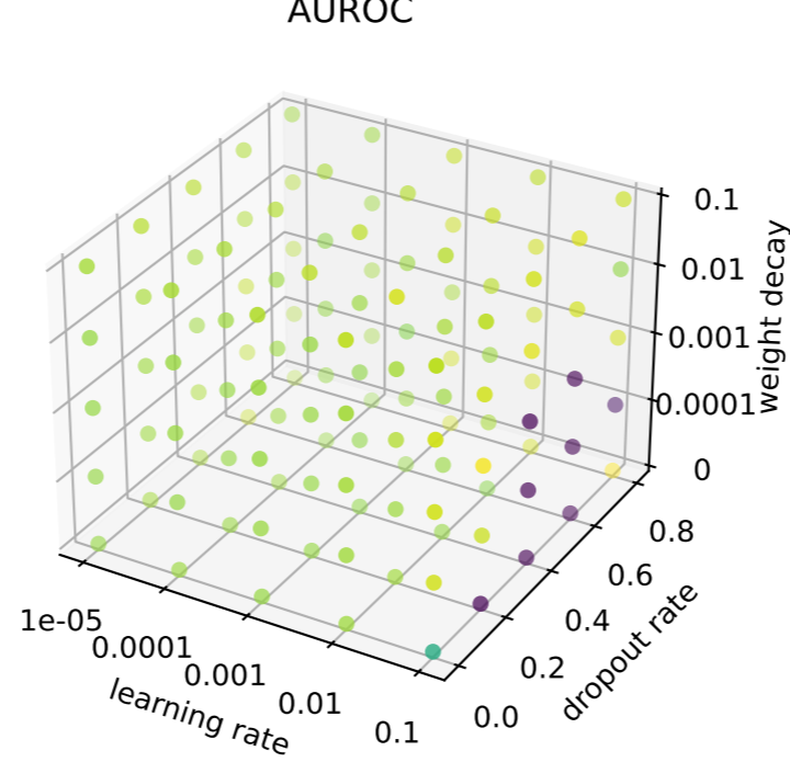
AUROC
