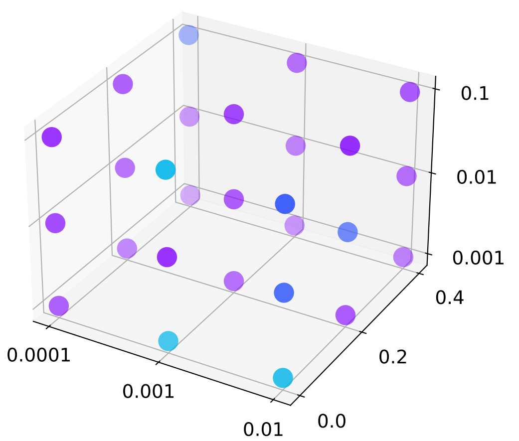
mDenseGCN
