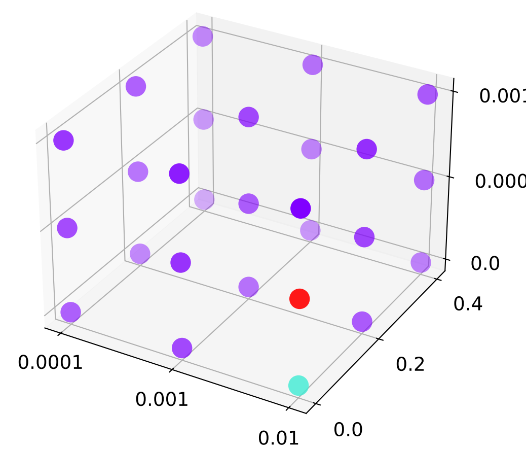
mGAT
