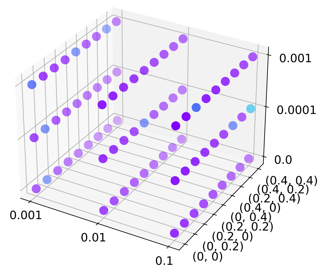
mDenseChebNet
