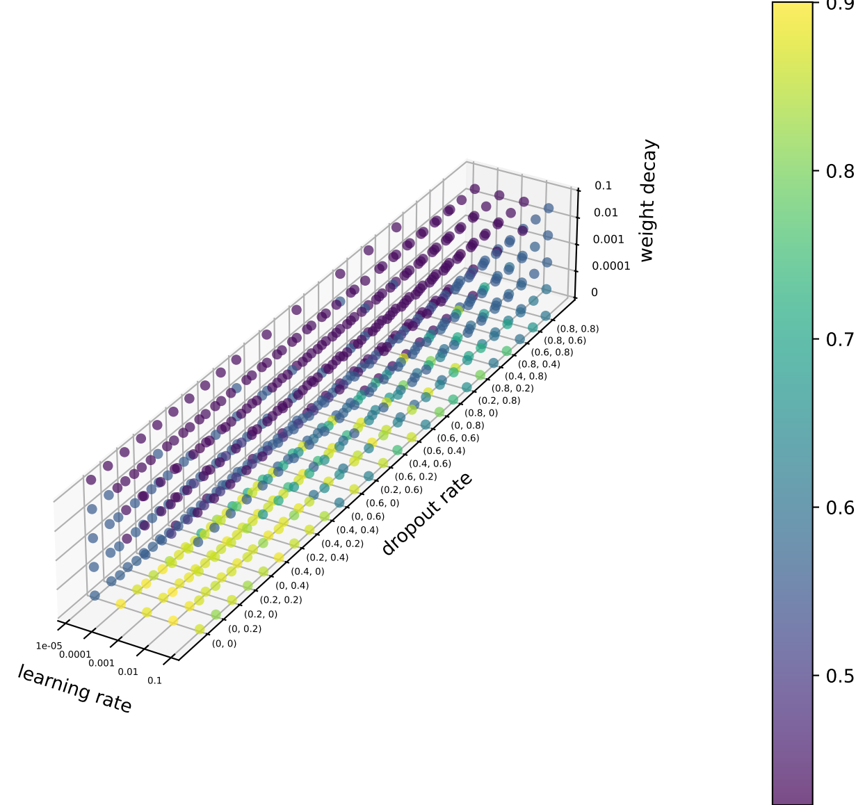
AUROC
