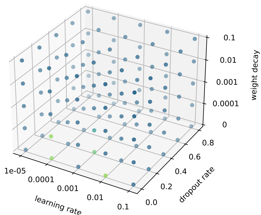
xGCN
