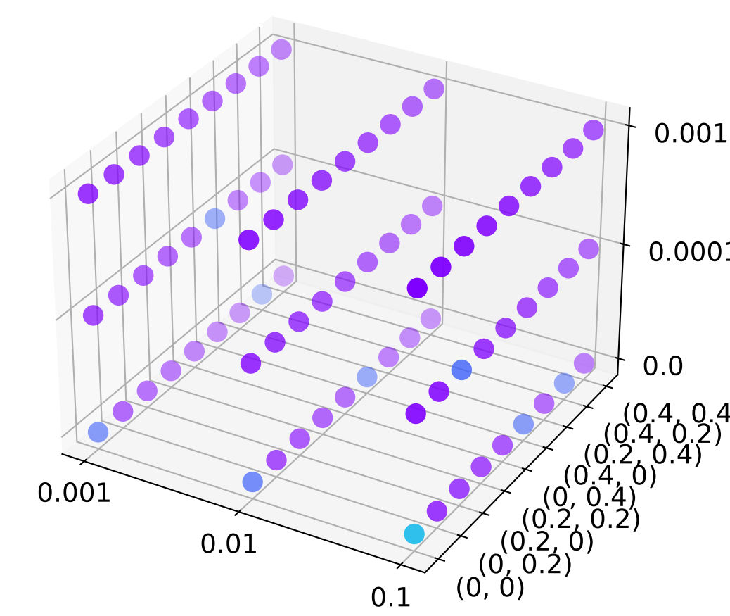
mChebNet
