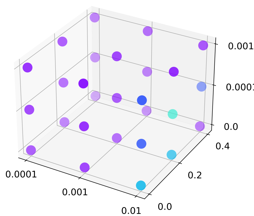
mResGAT
