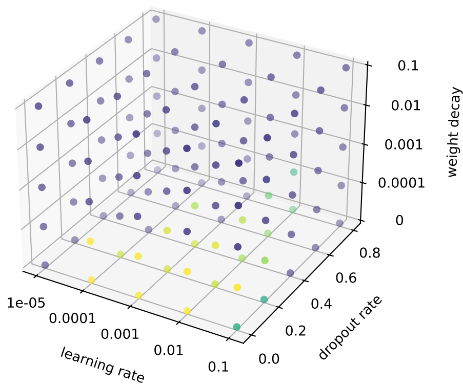
mGAT
