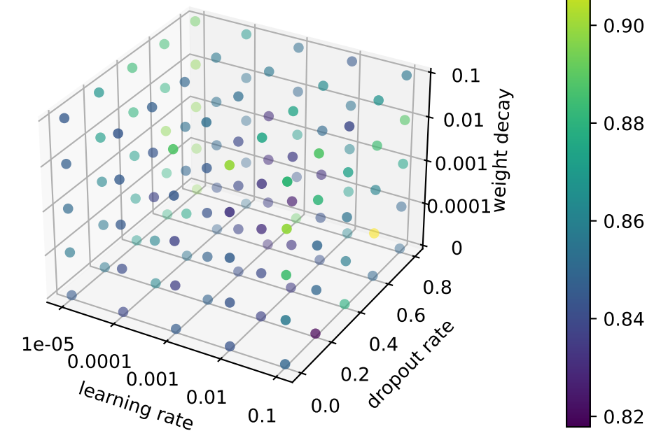
AUPRC
