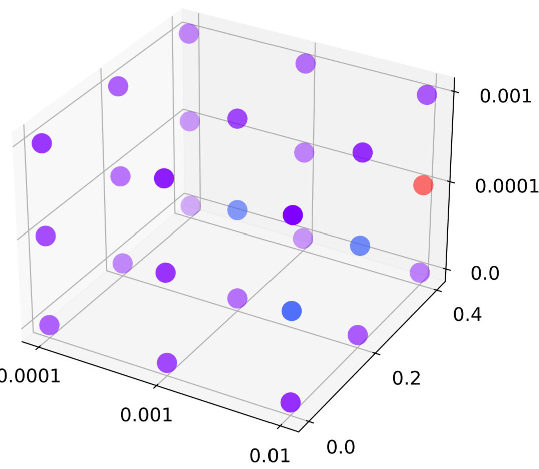
DenseGCN
