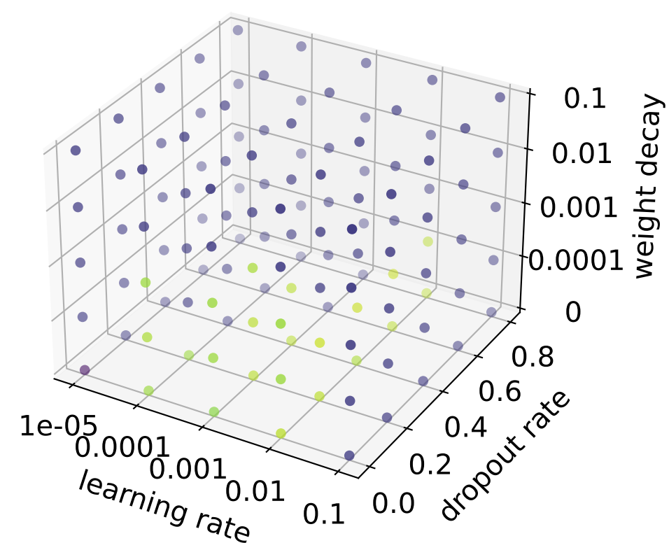
xChebNet
