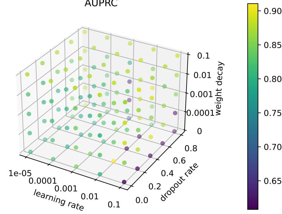
AUPRC
