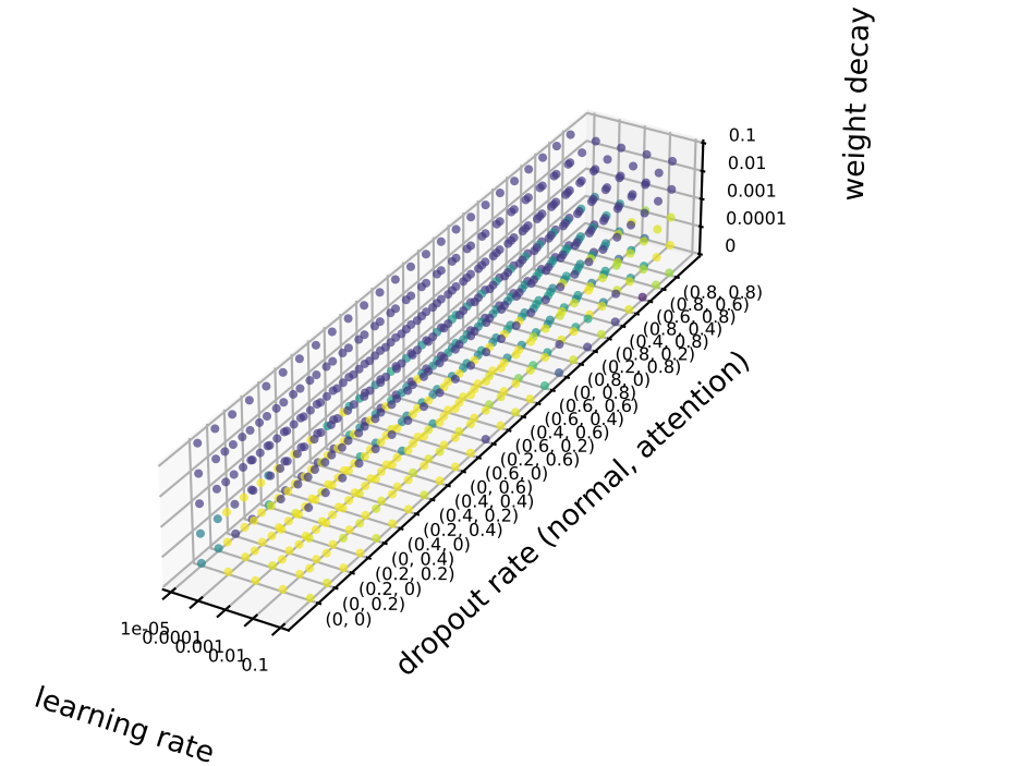
mDenseGAT
