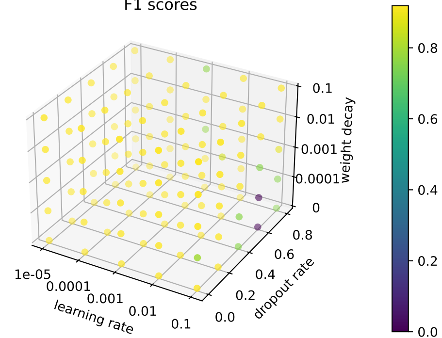
F1 scores
