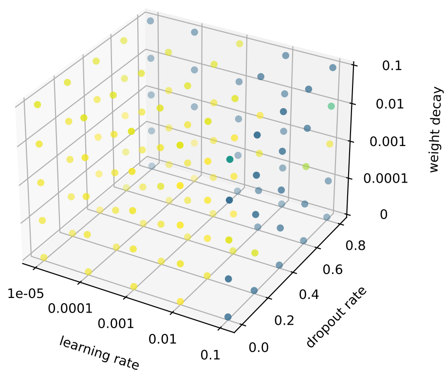
xMLP
