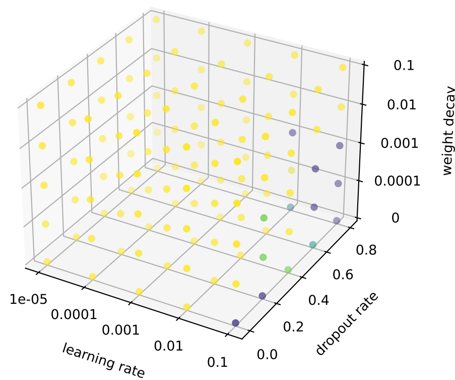
mResGCN
