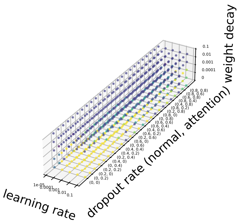
DenseGAT
