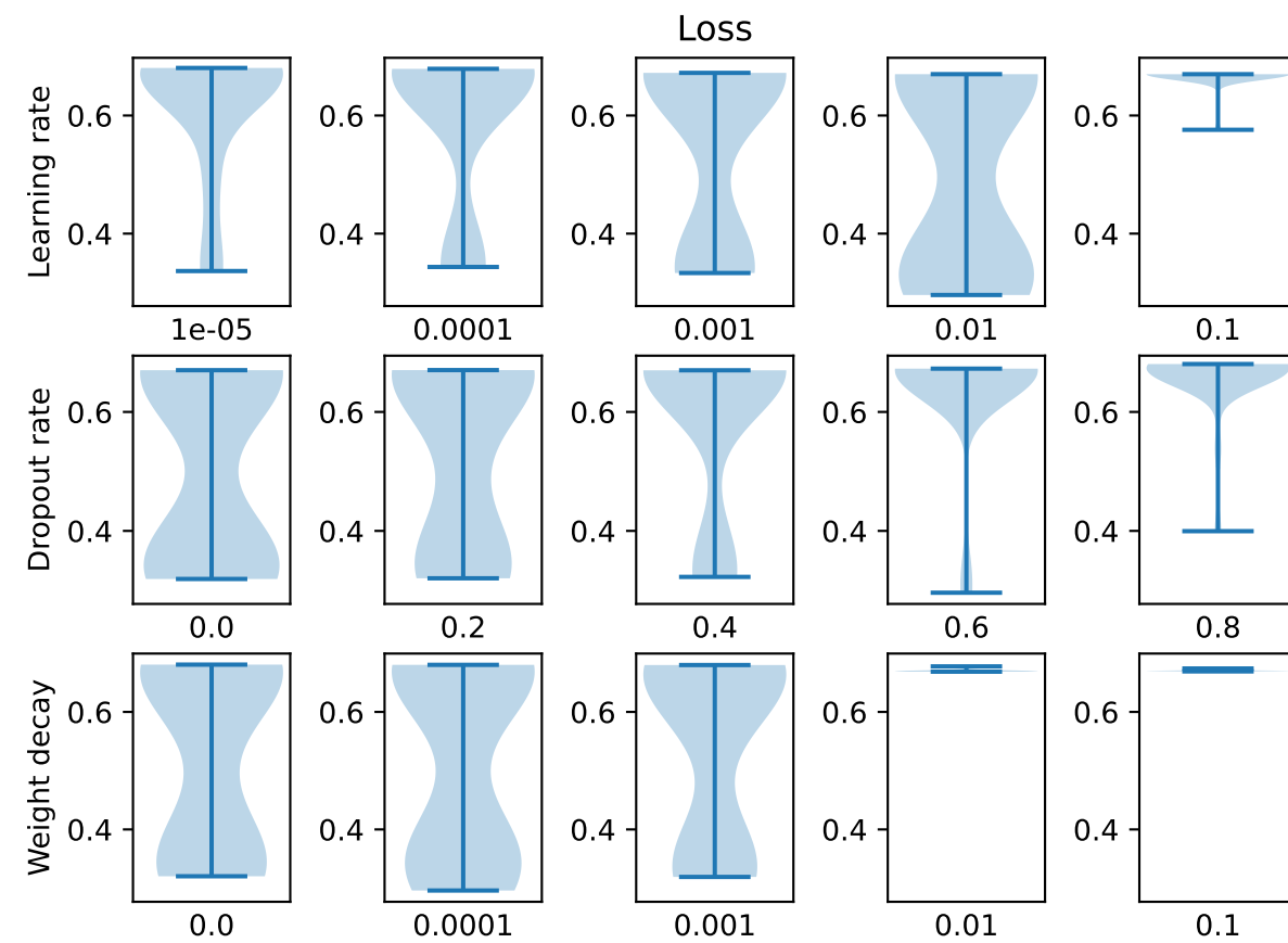
ResGCN (depth 7)
