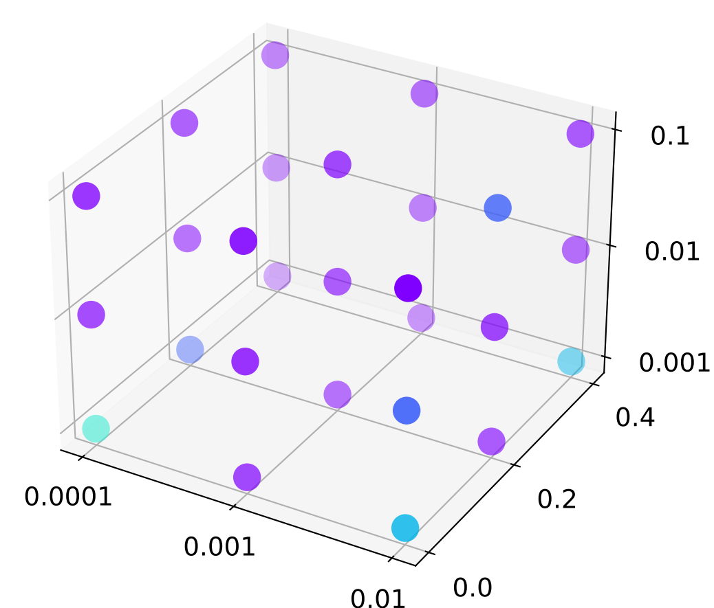
mGAT2MLP
