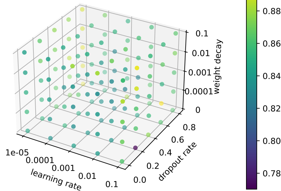
AUROC
