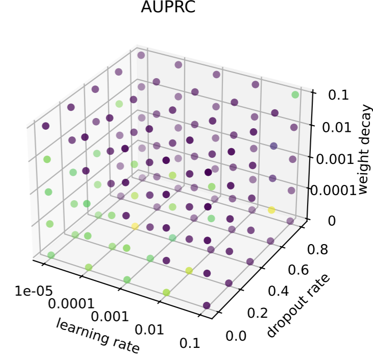
AUPRC
