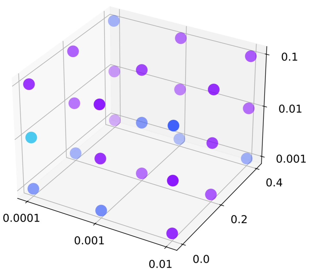
ResMLP
