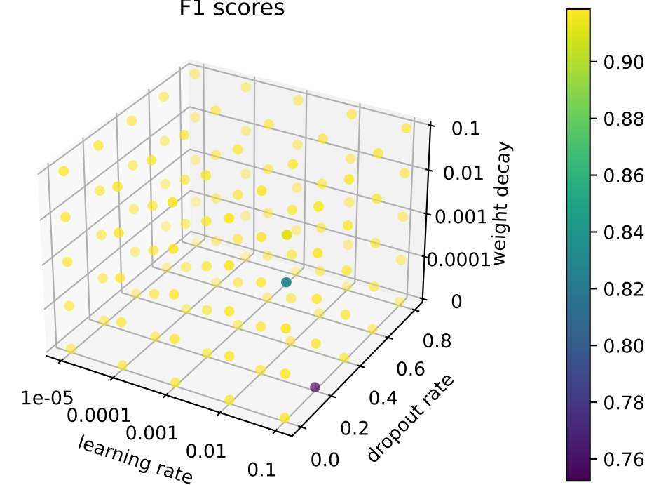
F1 scores
