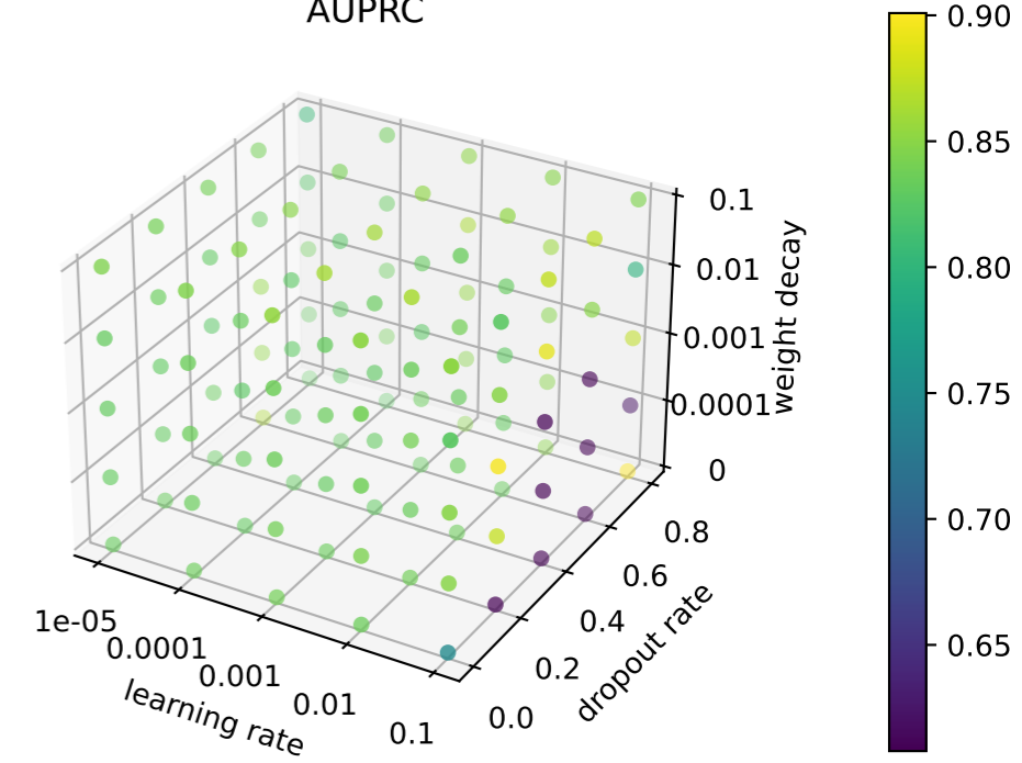
AUPRC
