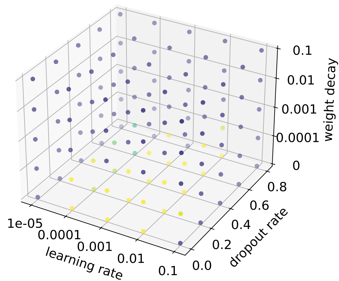
GCN
