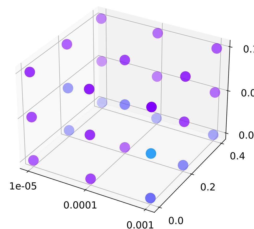
xResGCN
