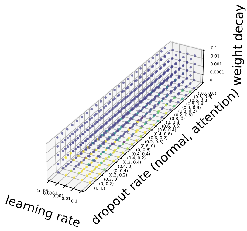
GAT
