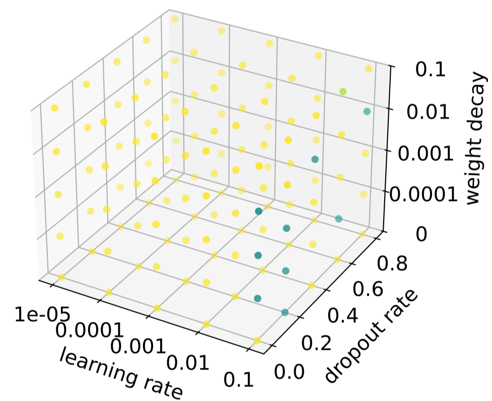
mDenseGCN2MLP
