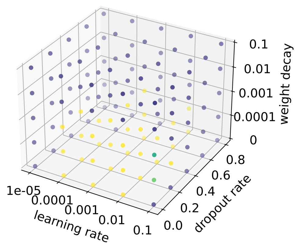
ResGCN
