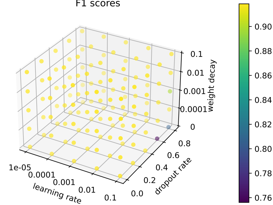
F1 scores
