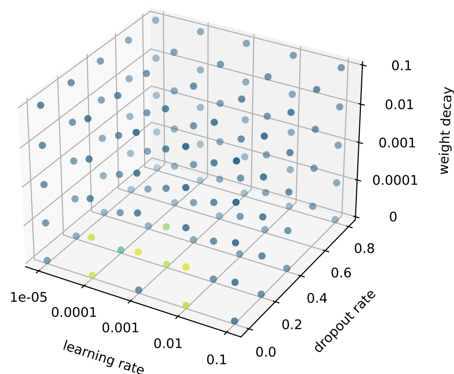
xDenseGCN
