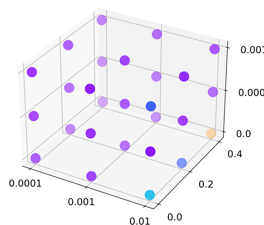
mGCN2MLP
