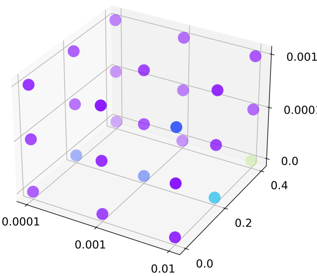
ChebNet
