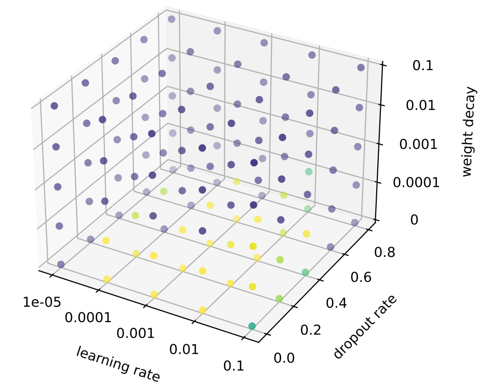
mDenseGAT
