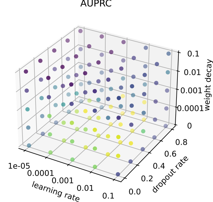
AUPRC
