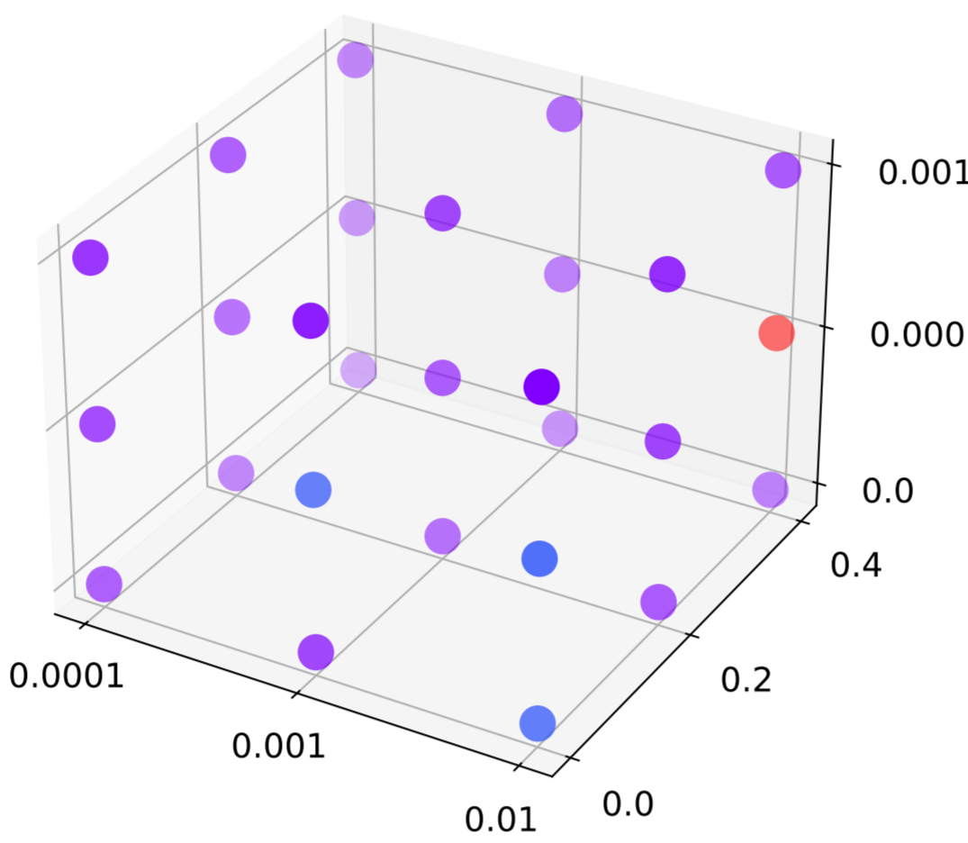
ResGCN
