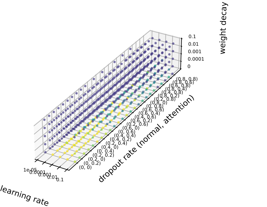
mGAT
