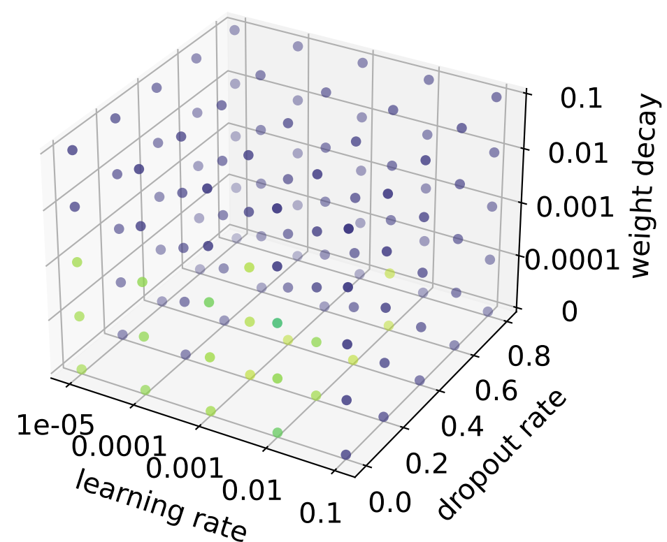
xResChebNet
