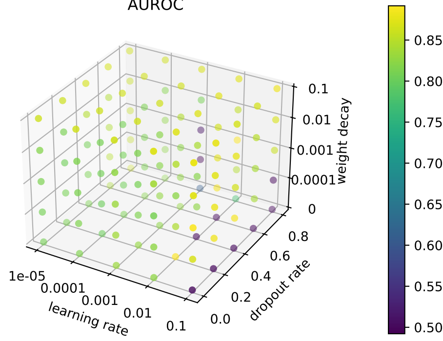
AUROC
