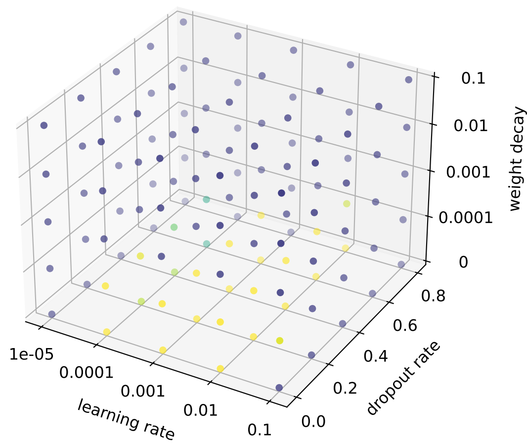
GCN
