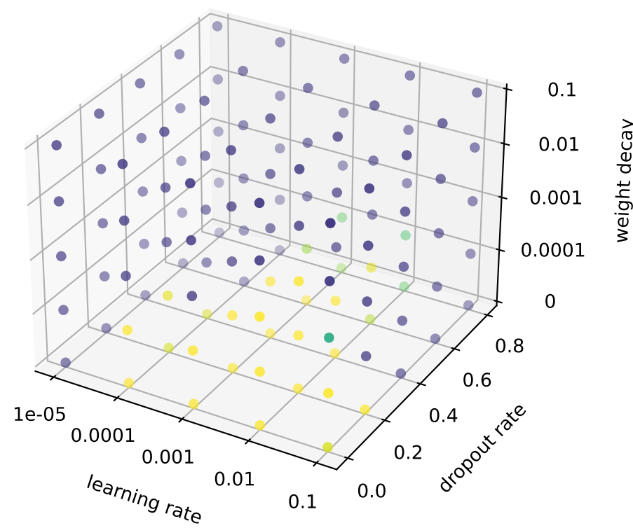
mResGAT
