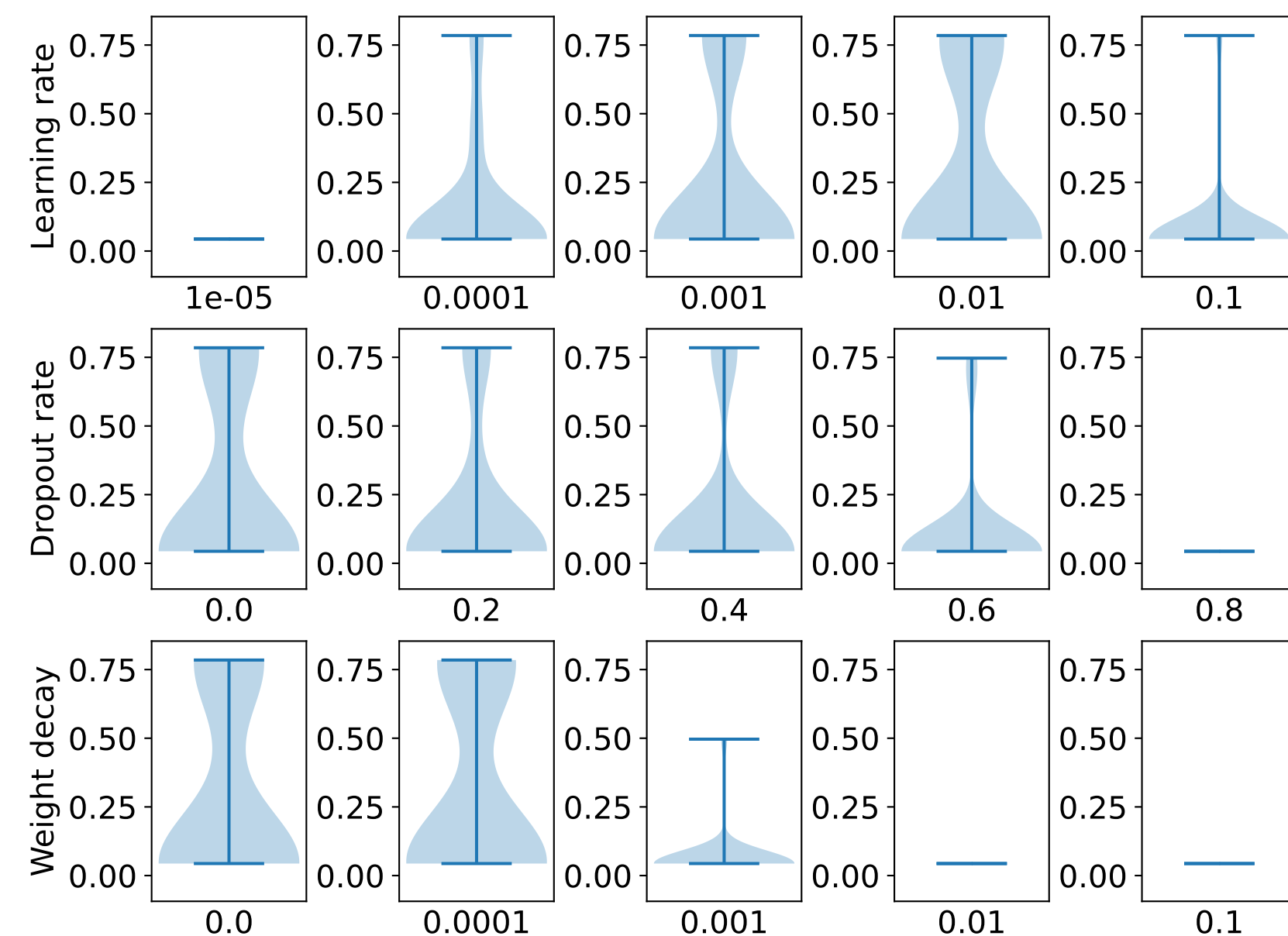
LightGAT
