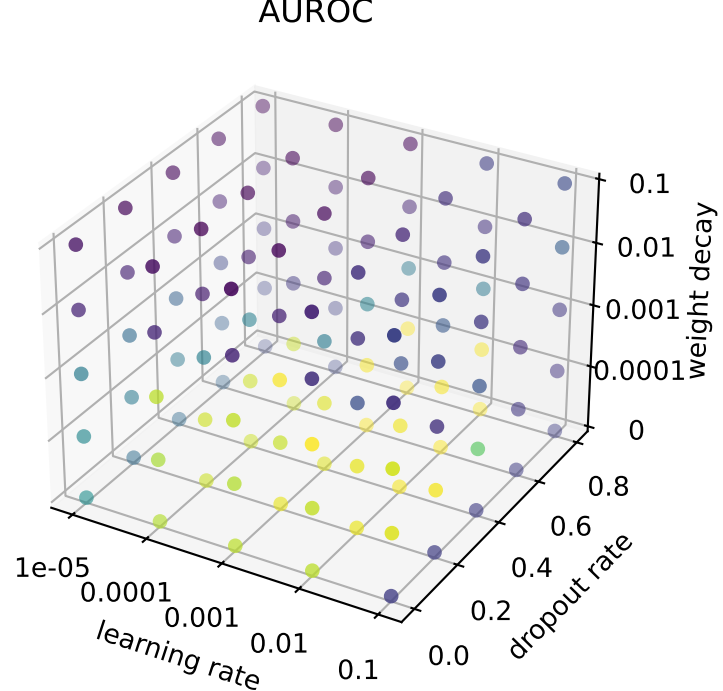
AUROC
