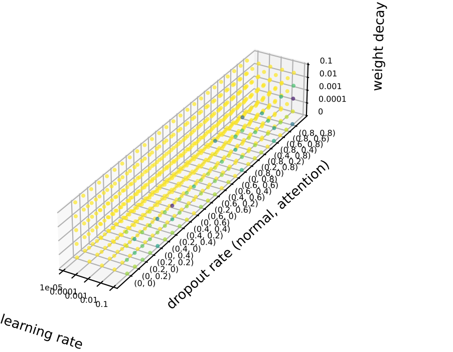
mGAT2MLP
