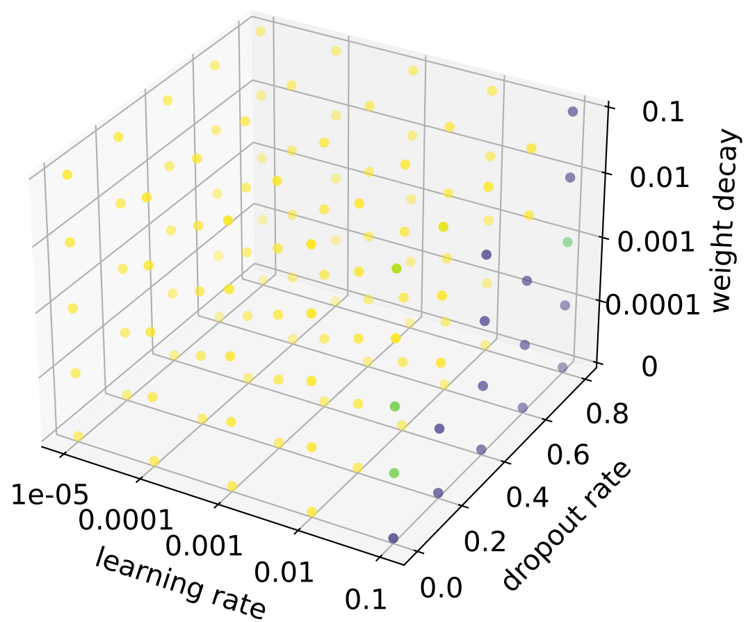
MLP
