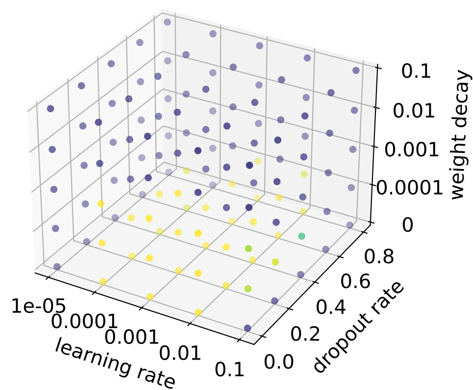
DenseGCN
