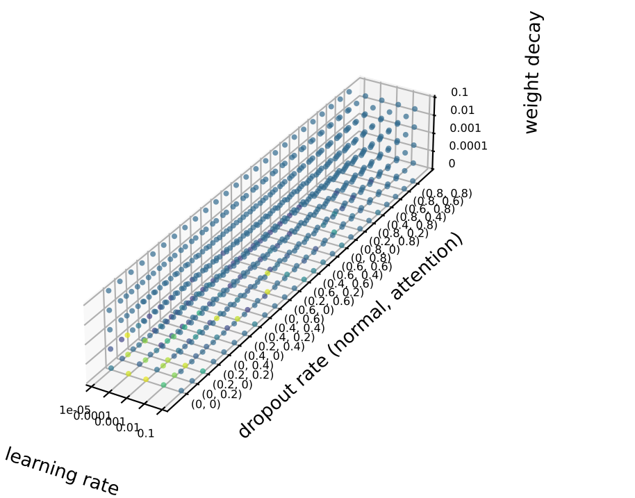
xResGAT
