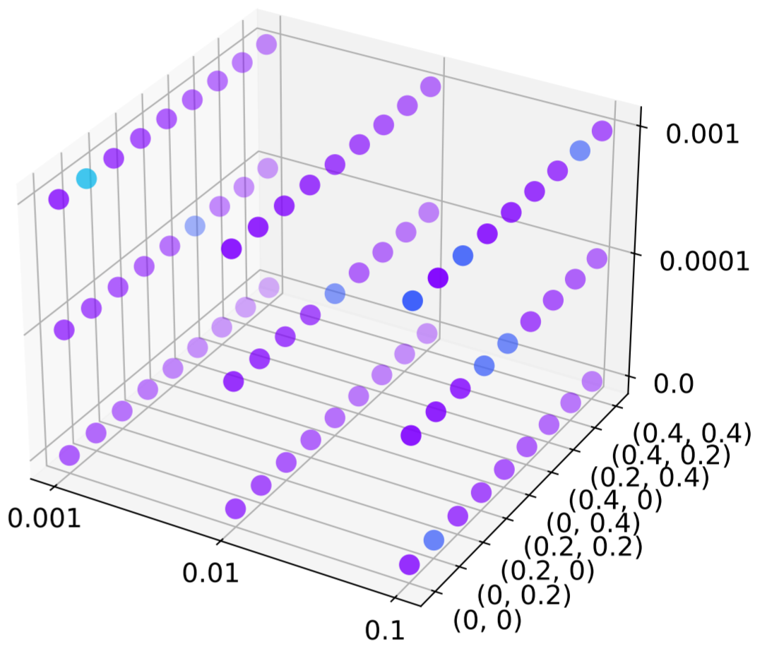
DenseGAT
