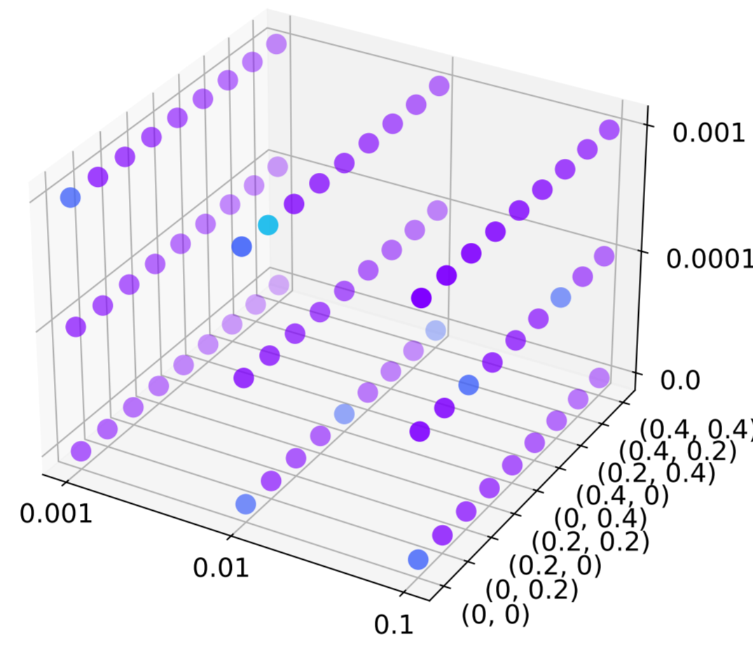
ResGAT
