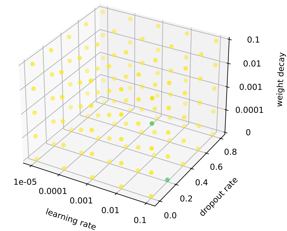
mDenseGCN
