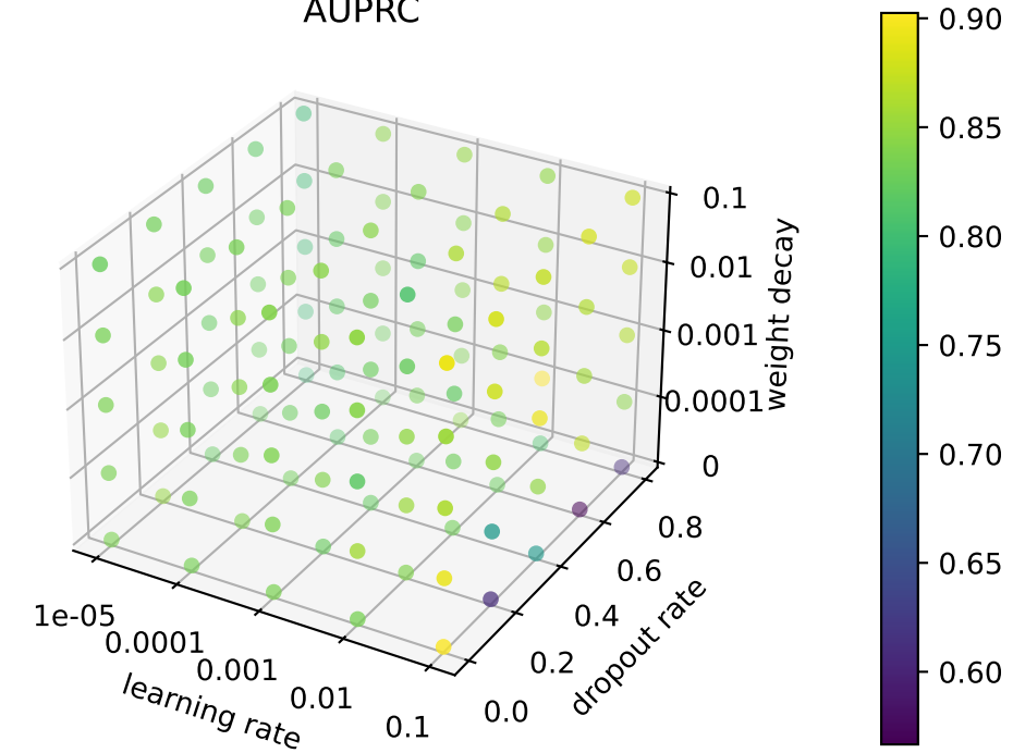
AUPRC
