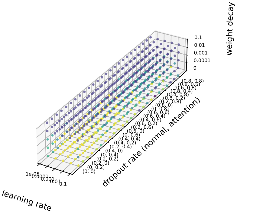
mResGAT
