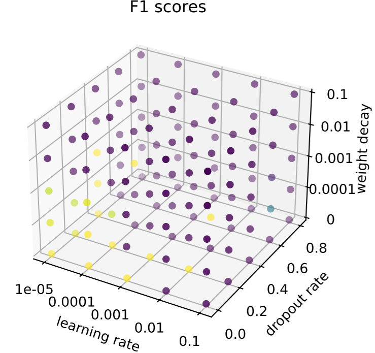
F1 scores
