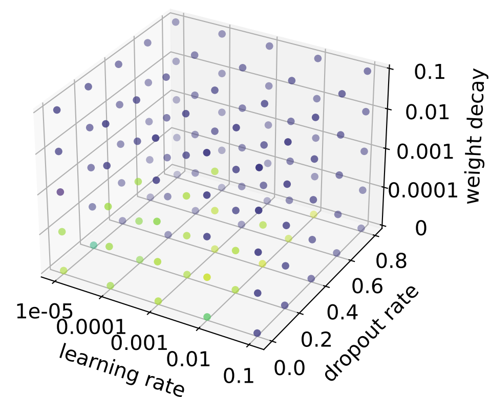
xDenseChebNet
