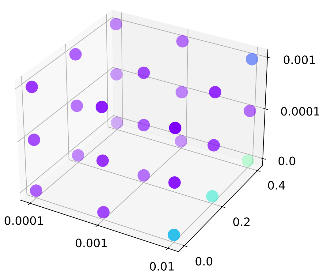
mDenseGCN2MLP
