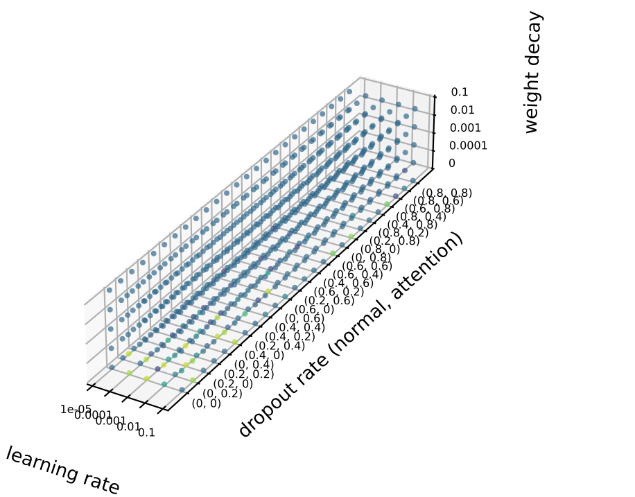
xDenseGAT
