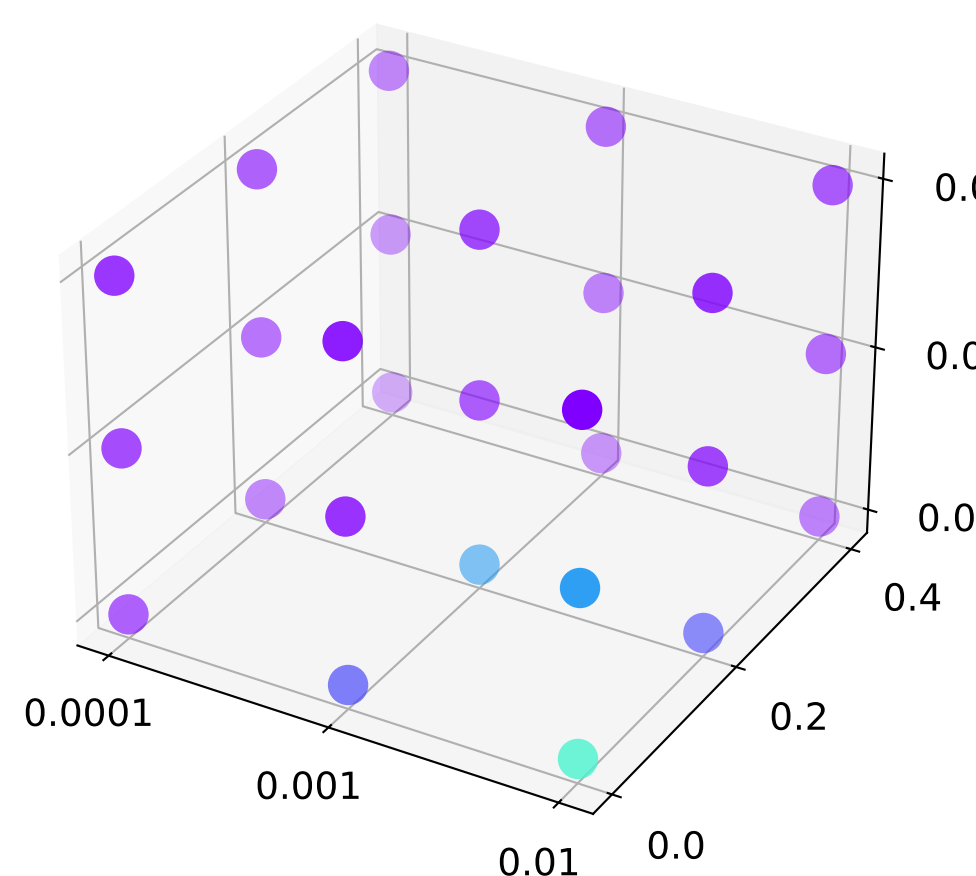
xResGAT
