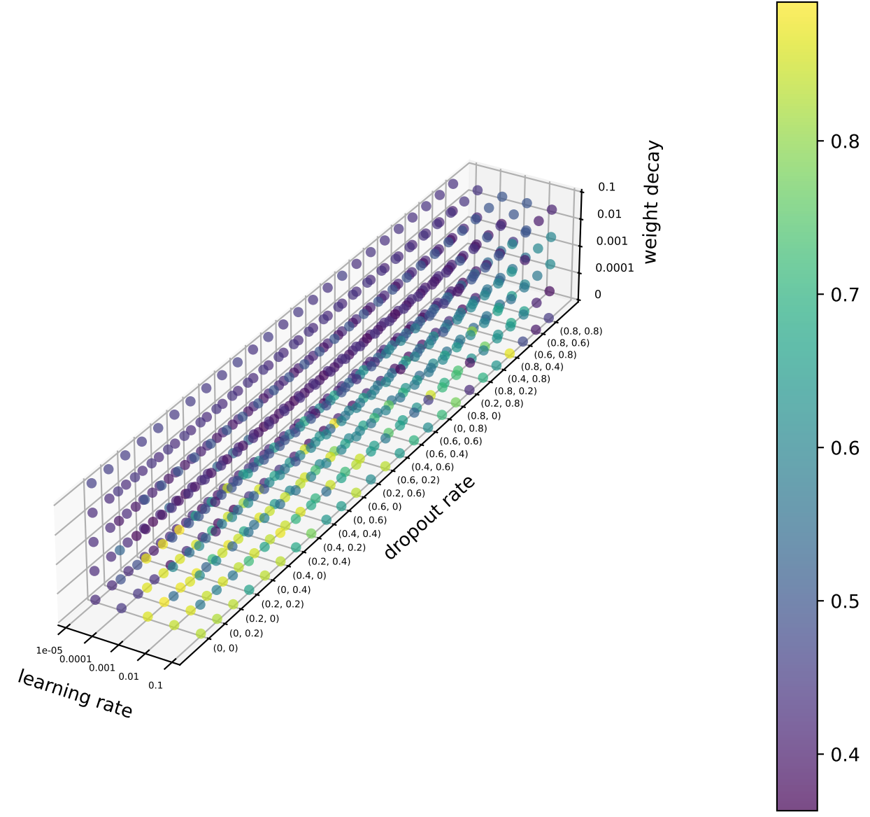
AUROC
