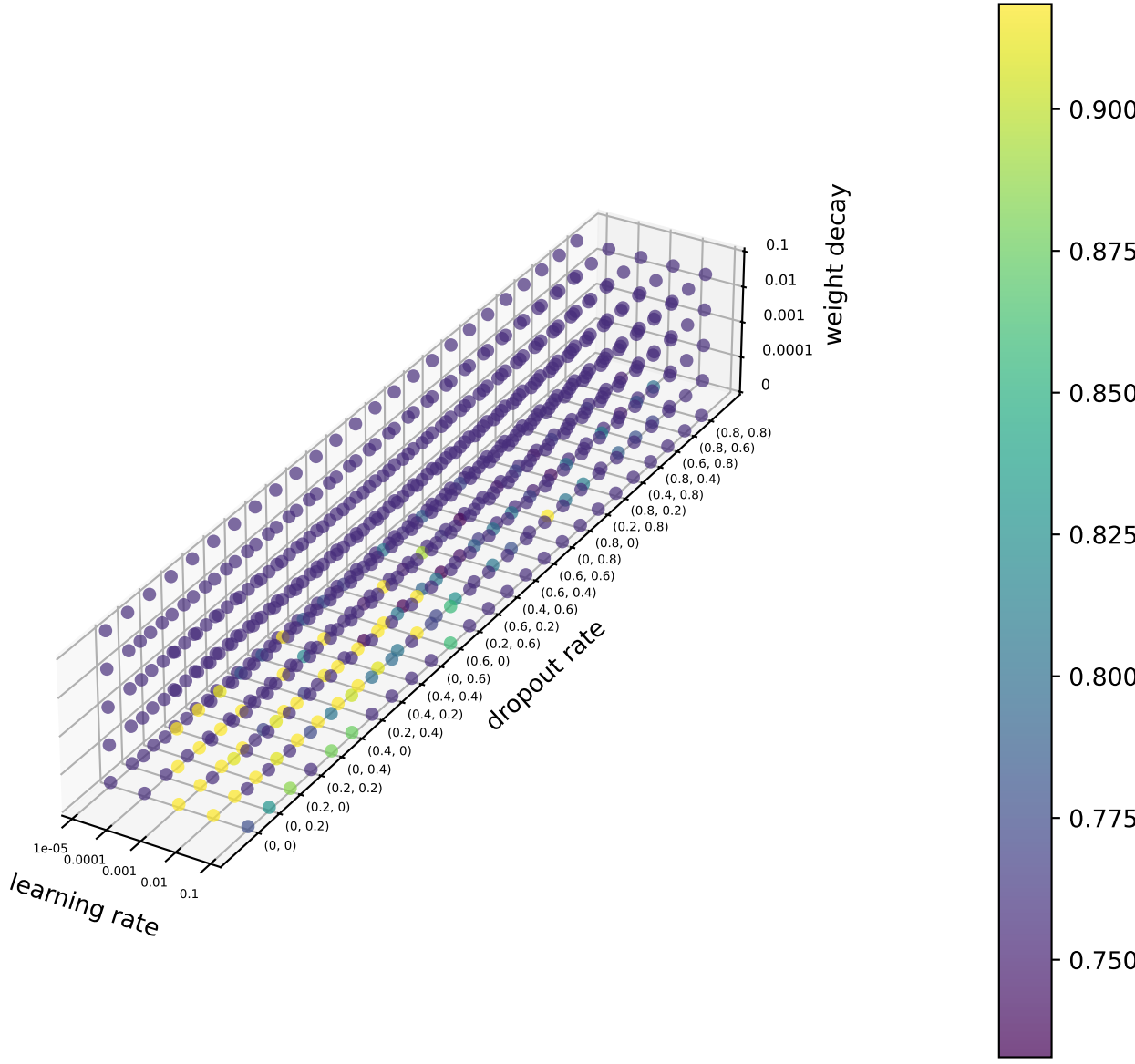
F1 scores
