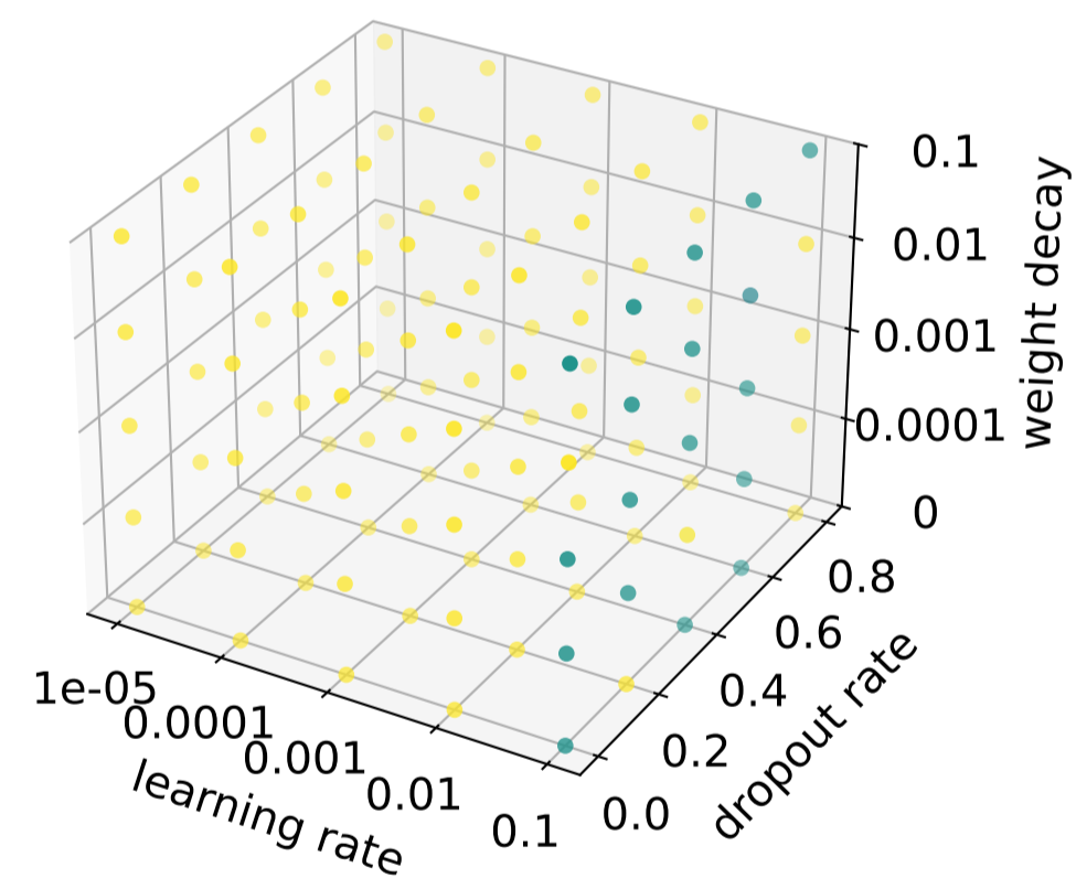
mGCN2MLP
