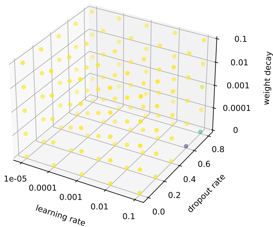
mGCN
