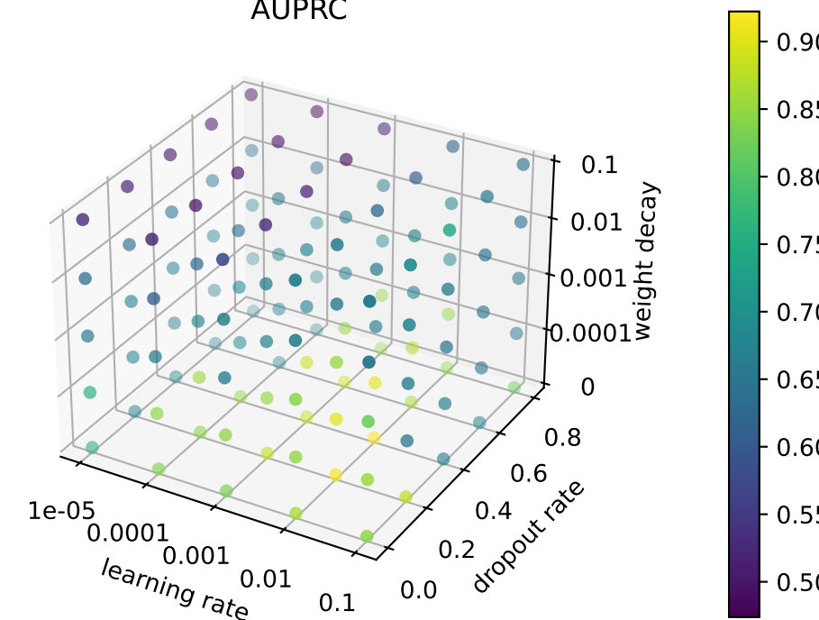
AUPRC
