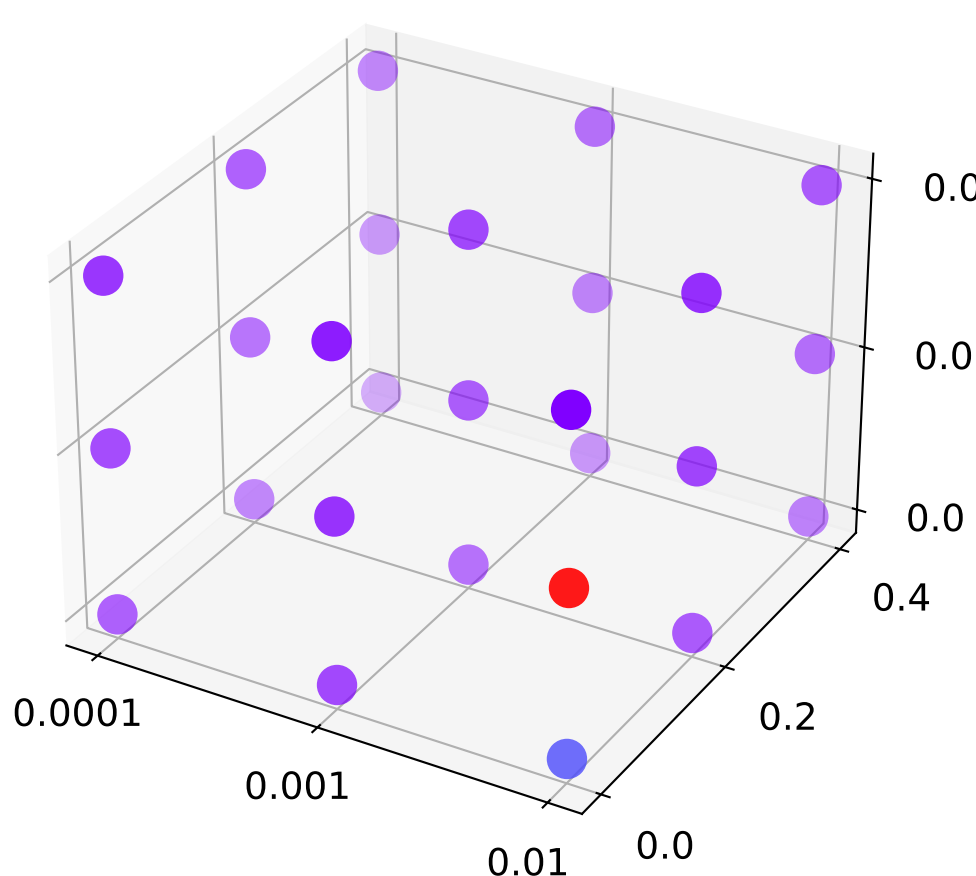
xDenseGAT
