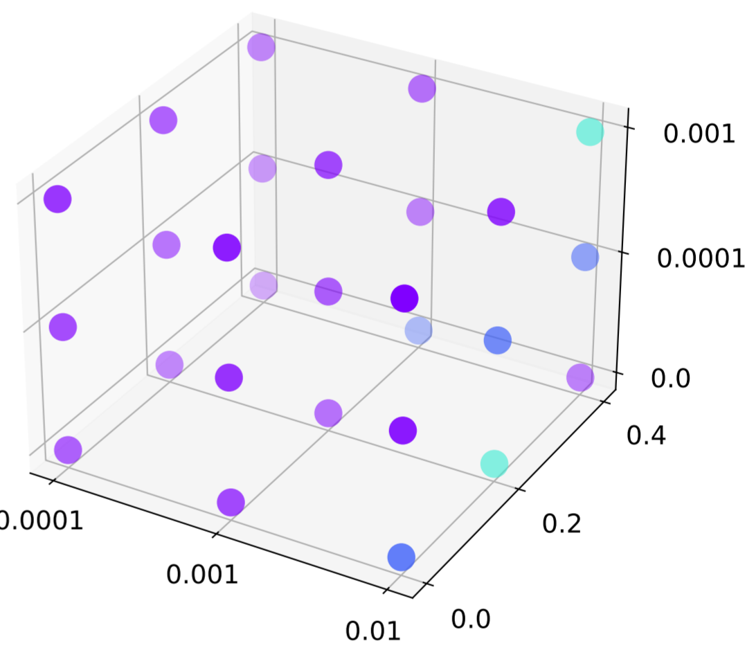
DenseChebNet
