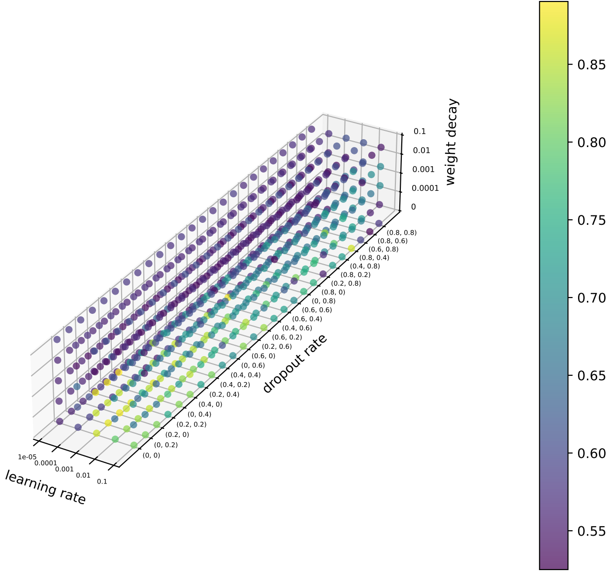
AUPRC
