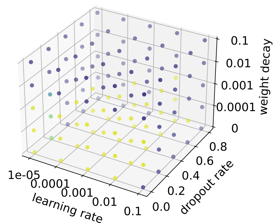
mChebNet
