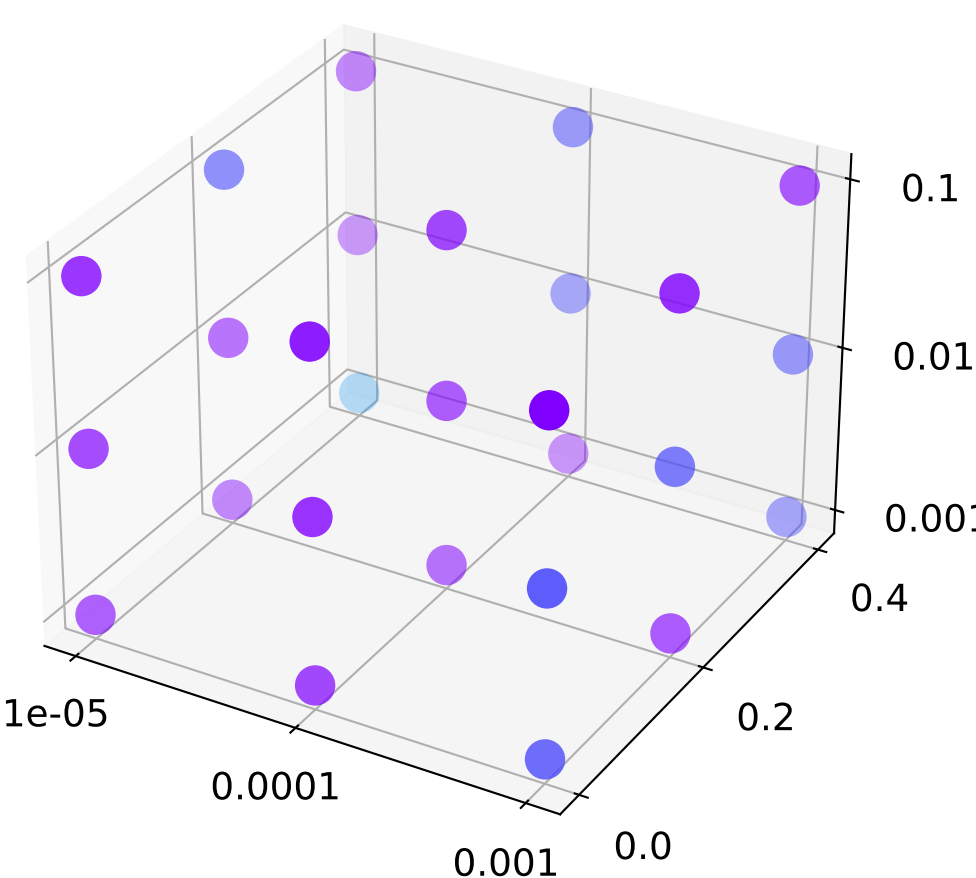
xGCN
