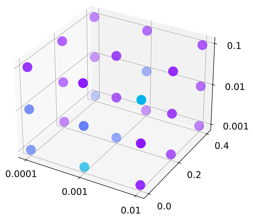
mResGCN
