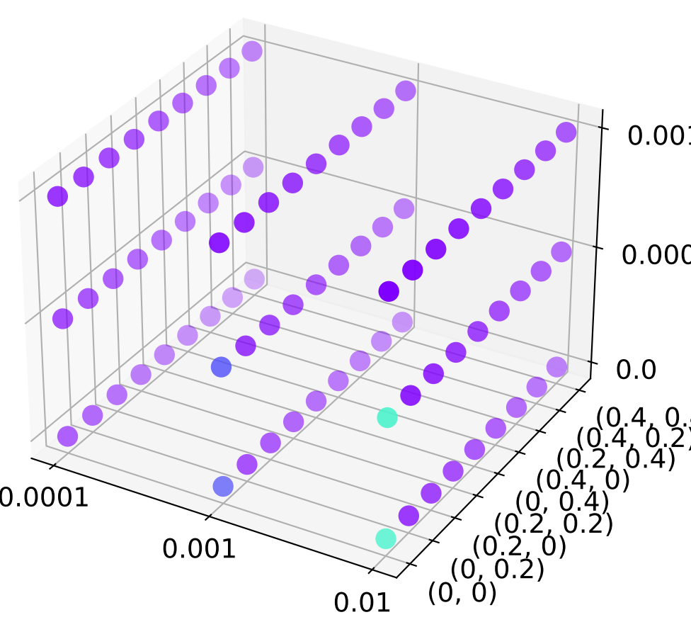
xChebNet
