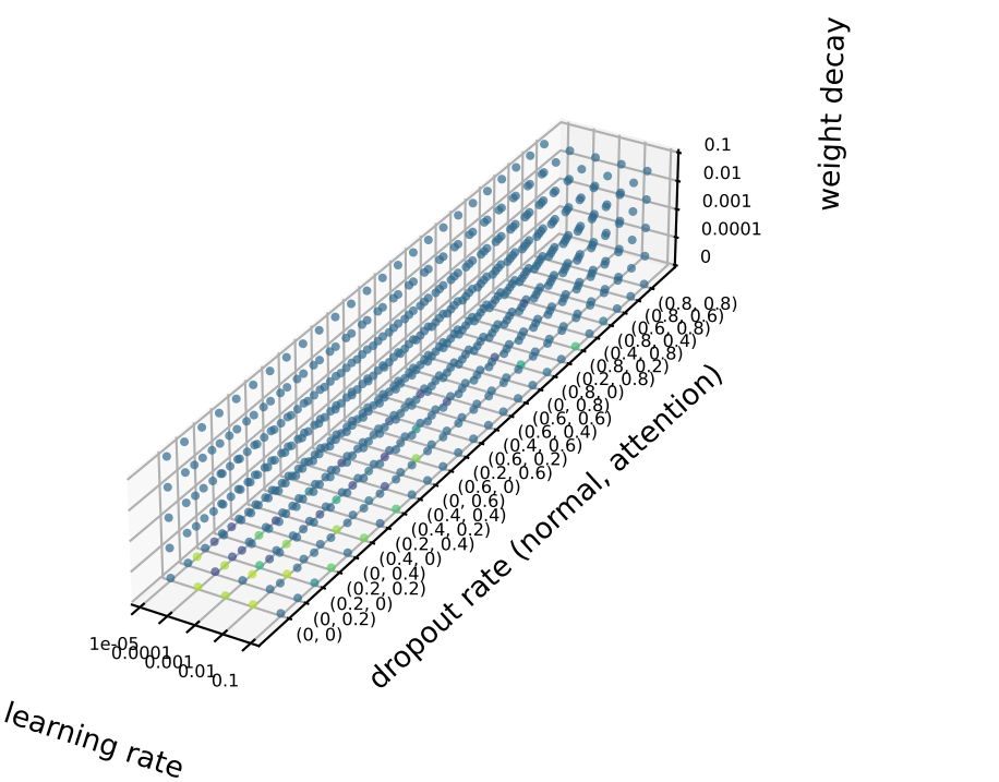
xGAT
