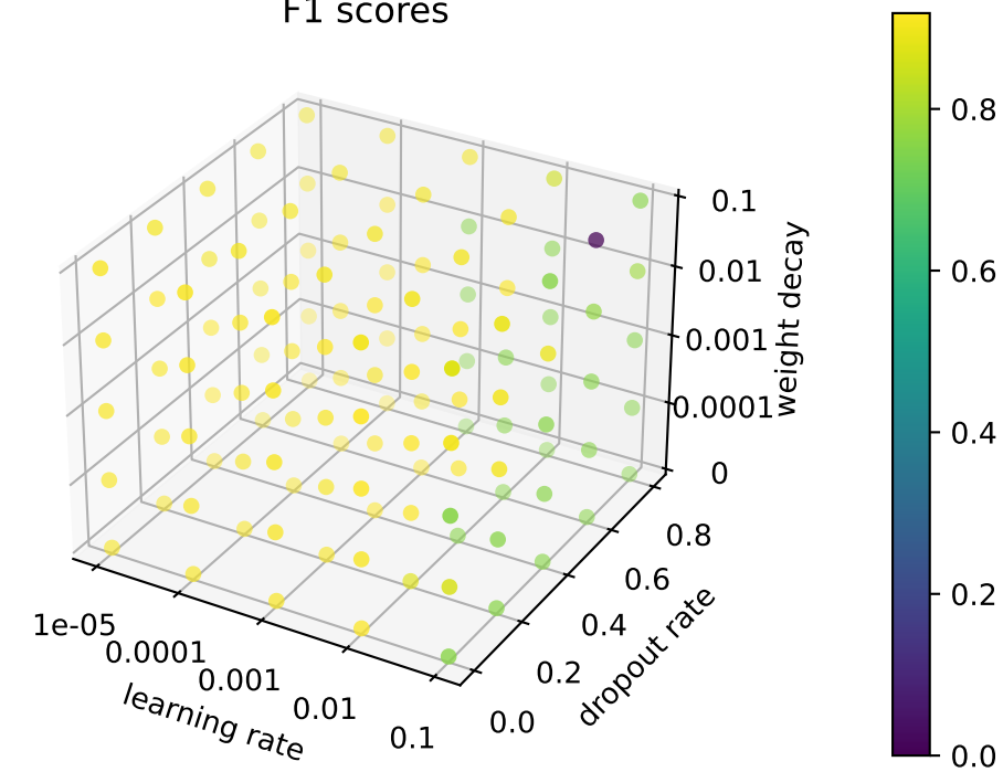
F1 scores
