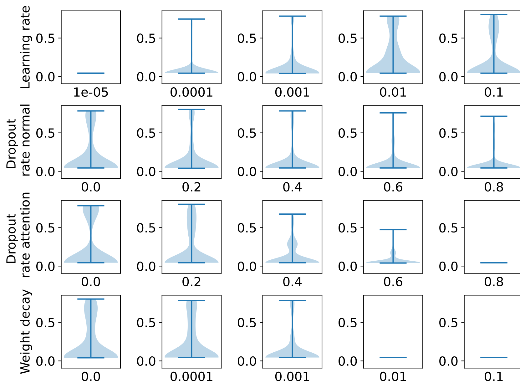
LightGAT
