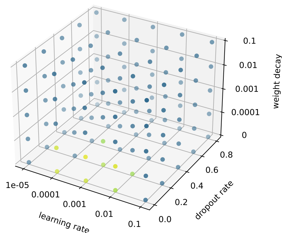
xResGCN
