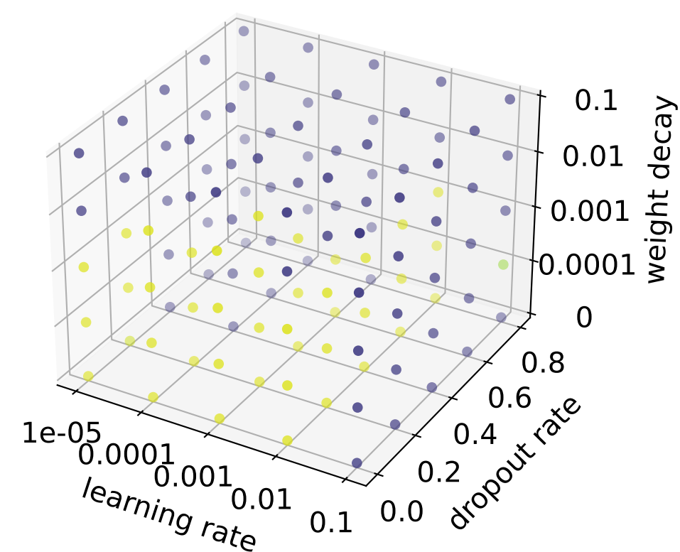
DenseChebNet
