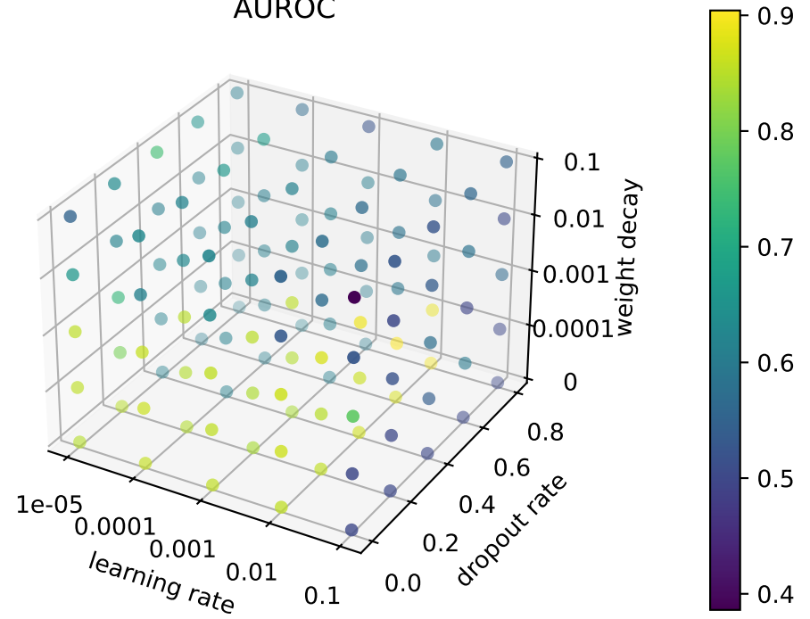
AUROC
