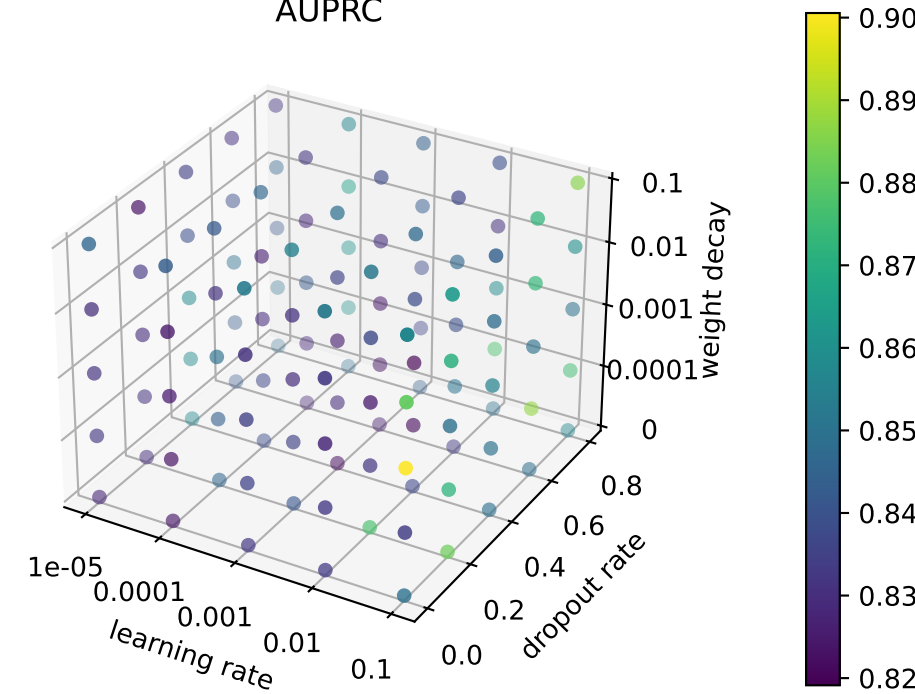
AUPRC
