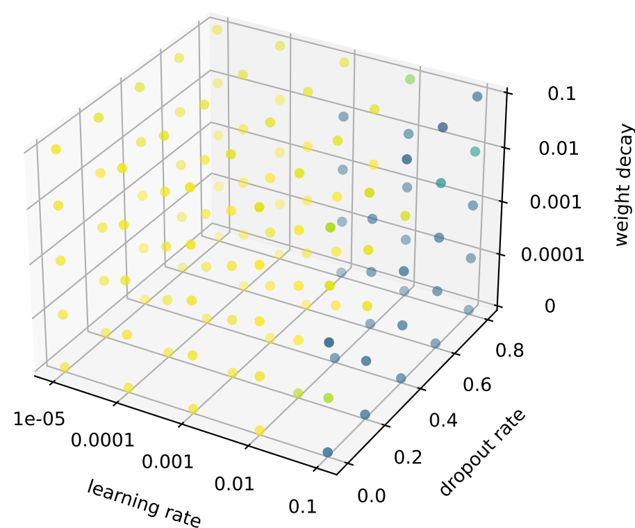
xResMLP
