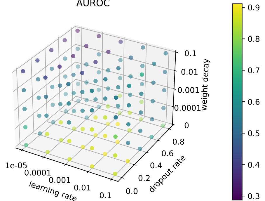
AUROC
