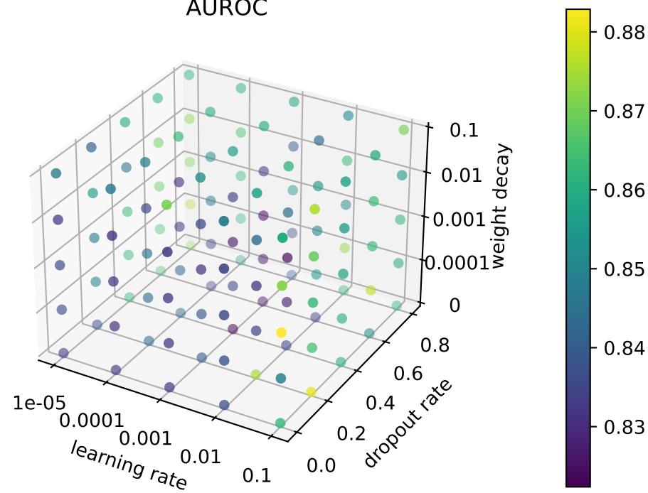
AUROC
