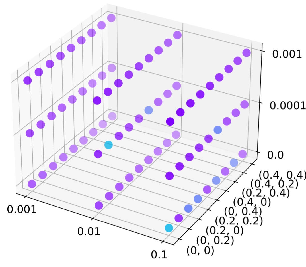
GAT
