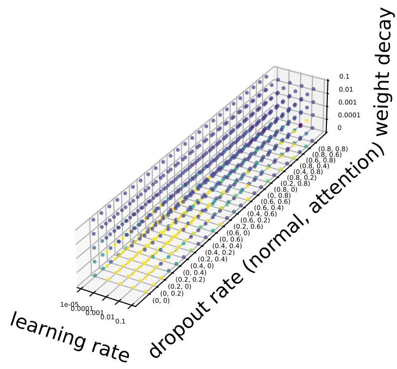
ResGAT
