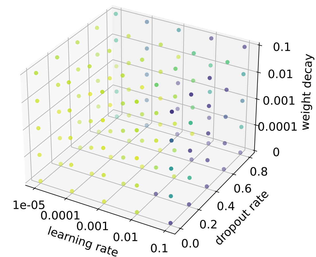
MLP
