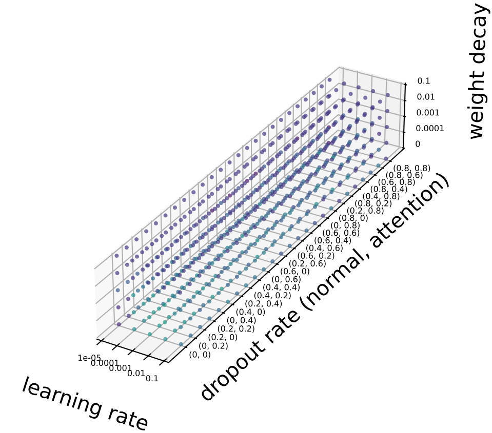
GAT
