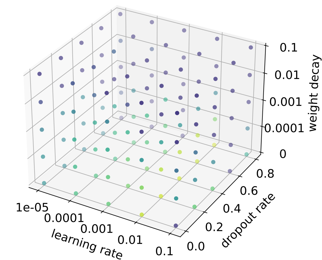
ChebNet
