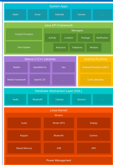
Архитектура Android
