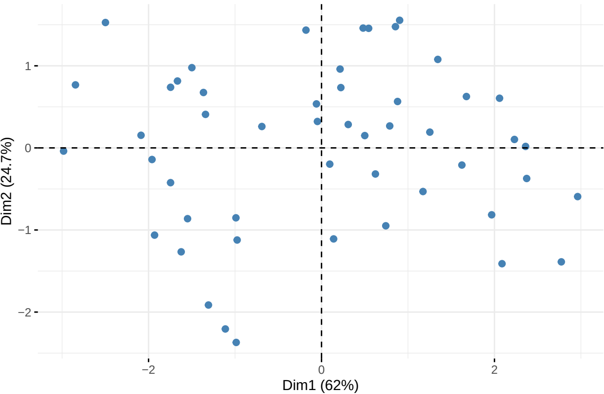
Score plot: individuos en el espacio PC1-PC2
