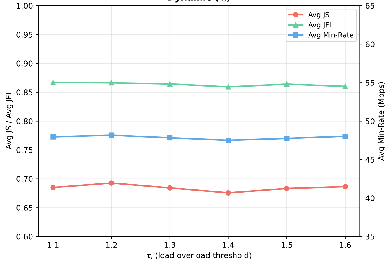
Dynamic ( \tau_l )
