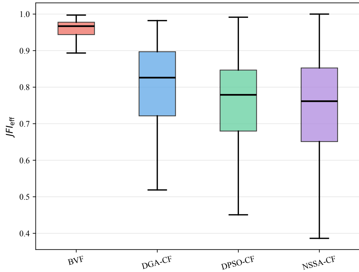
(a) JFI_eff 分布
