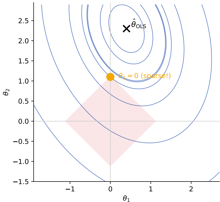
Lasso ( L_1 ): corner \Rightarrow \theta_1 = 0
