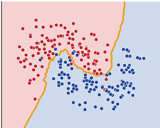
KNN (k=15): local
