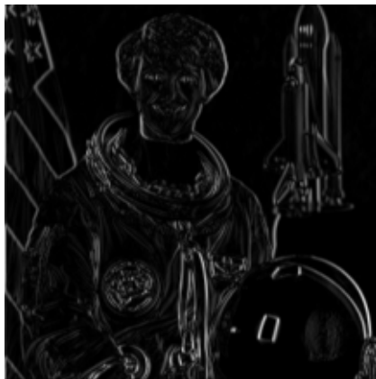
Sobel X
