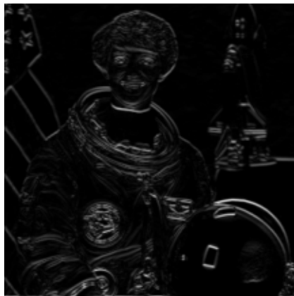
Sobel Y
