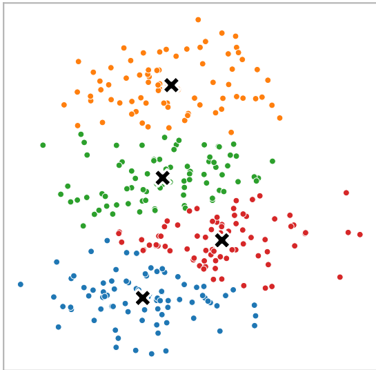
k-means++ inertia = 876
