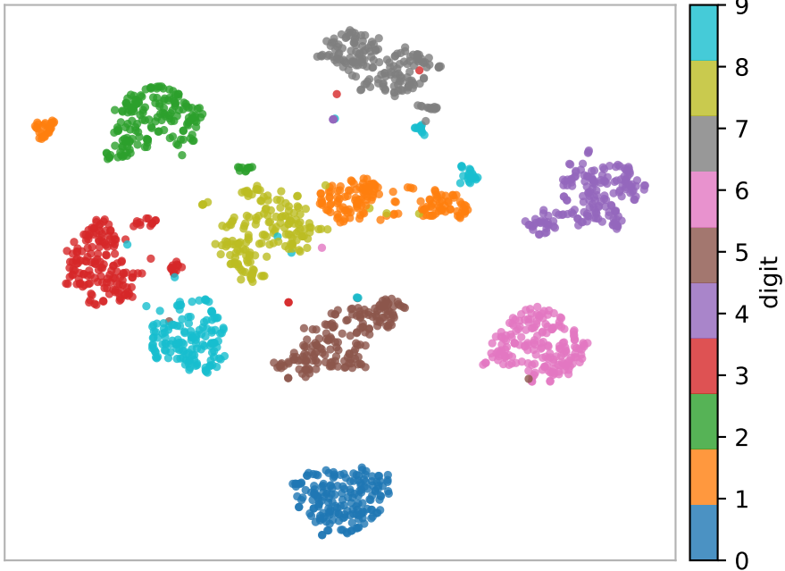
t-SNE of digits
