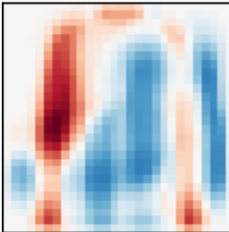
PC3 (6%)
