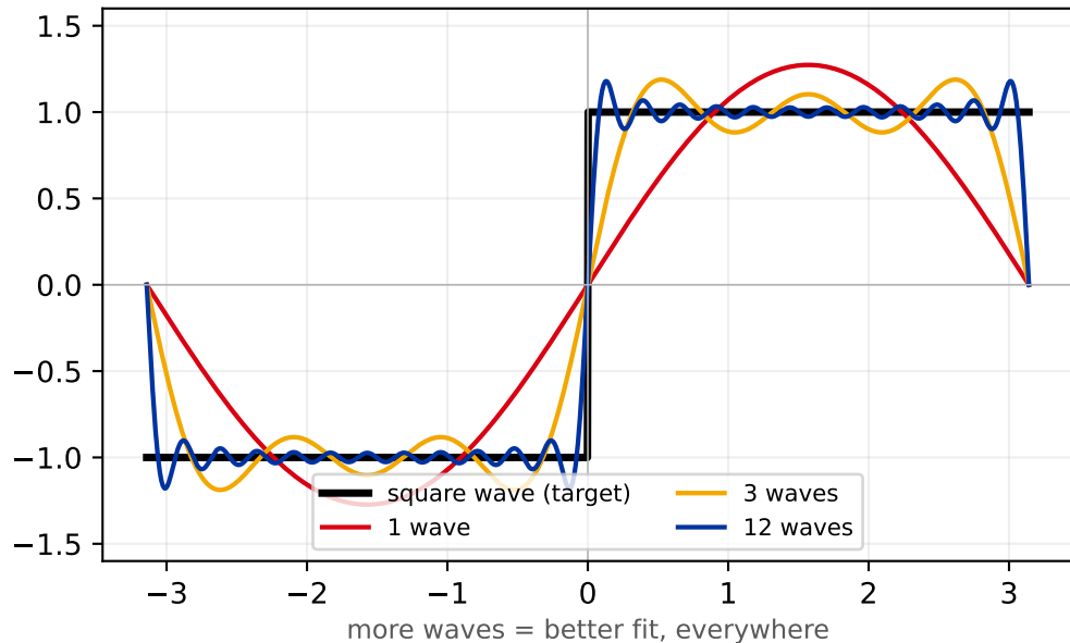
Fourier: sum of WAVES \sin x, \sin 3x, \dots
