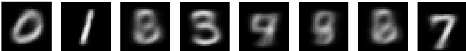
AE (2)
