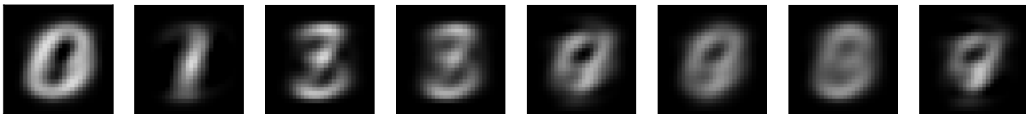
PCA (2)
