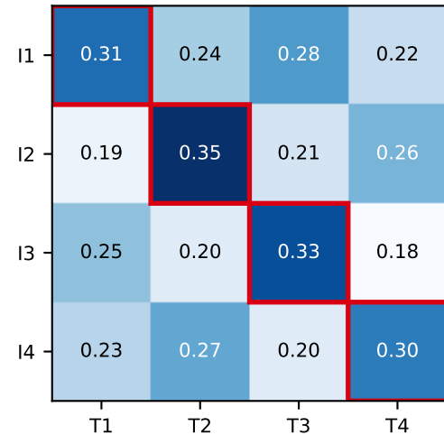
1. cosine similarities s_{ij}
