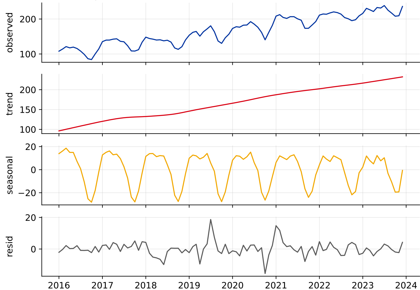
STL decomposition (statsmodels)
