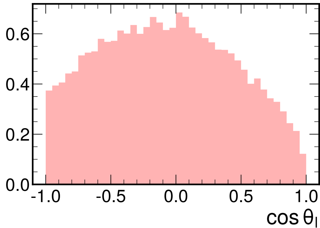
Asimetría Forward-Backward
