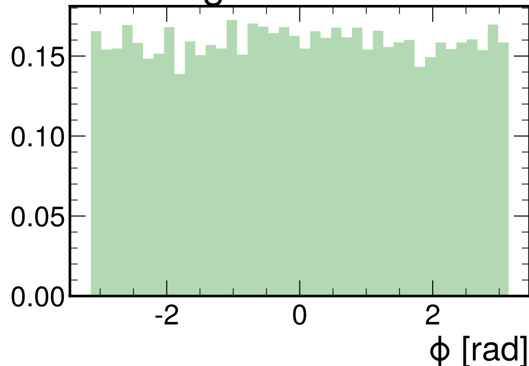
Ángulo Azimutal
