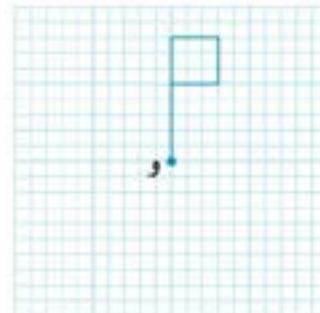
الرتبة 2
