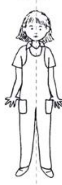
خط التماثل
