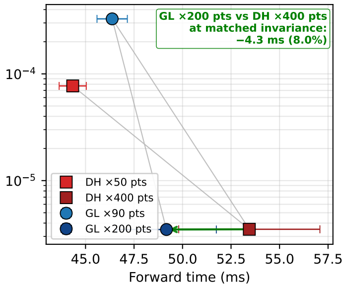
OC20 EqV2-31M (8L / 128ch / lmax=4 / mmax=2)
