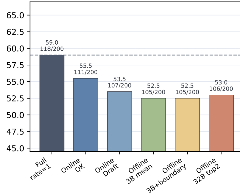
2wikimqa
