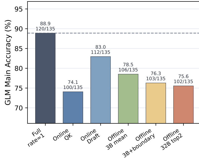
MuSiQue
