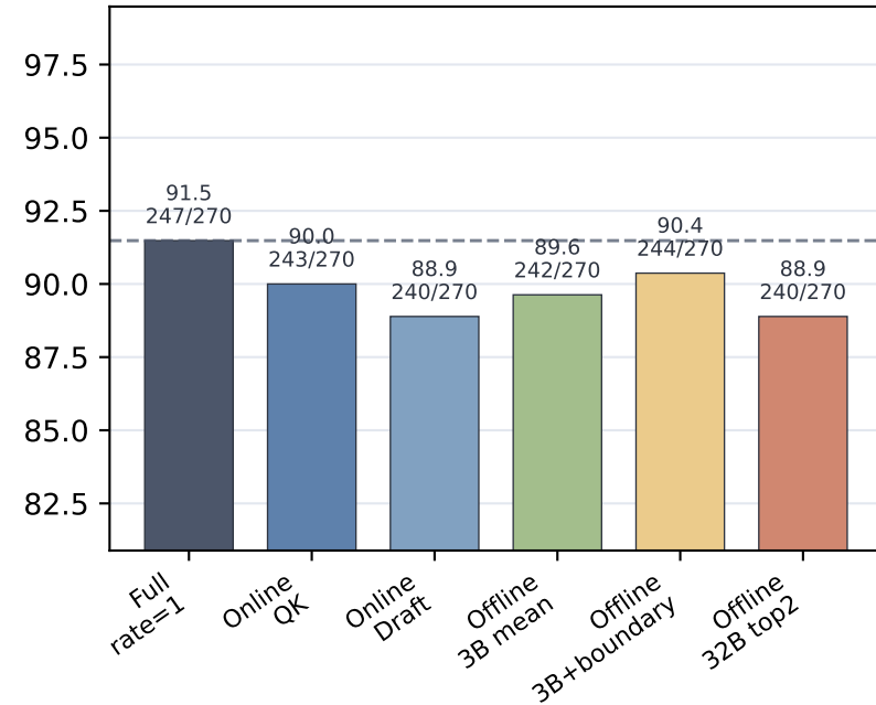
triviaqa
