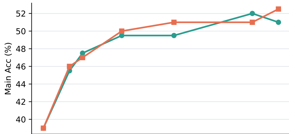
2WikiMQA
