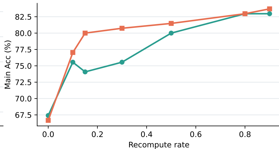
MuSiQue
