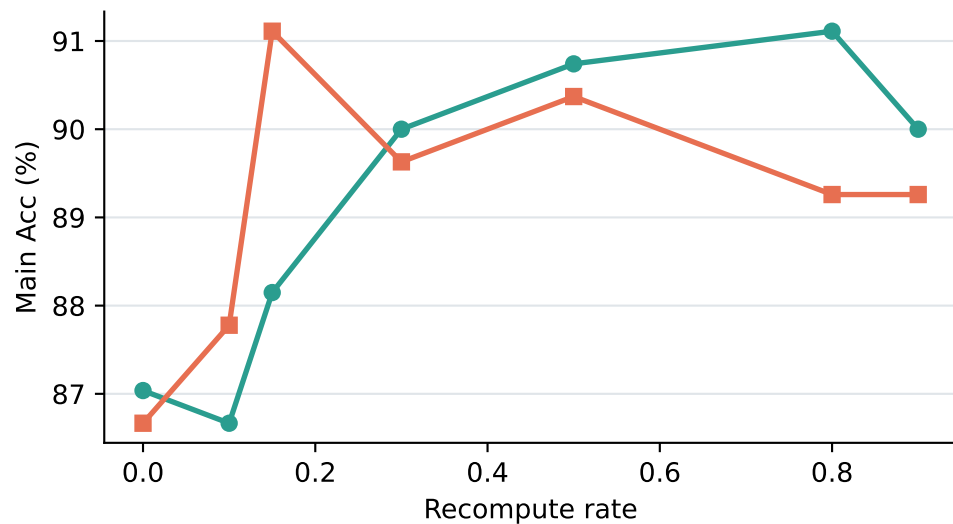
TriviaQA
