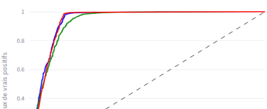
Courbes ROC
