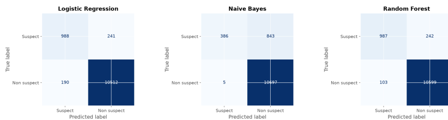
Matrices de confusion des 3 modèles classiques
