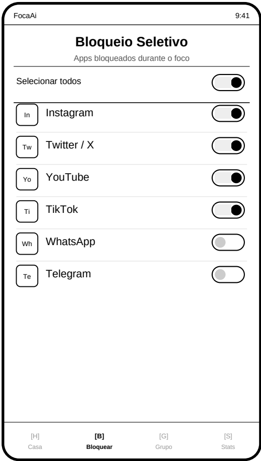
3. Bloqueio Seletivo
