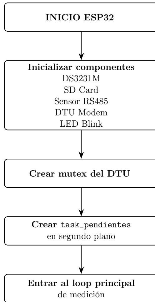
Figura 7: Secuencia inicial de ejecución del firmware en el ESP32.
