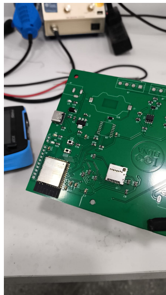
Figura 4: Inspección posterior al horneado de la PCB para verificar la calidad de las soldaduras y la correcta alineación de los componentes.
