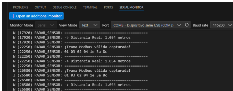
Figura 10: Lectura del sensor de nivel RS485 observada en el monitor serial. Se verifica la recepción de una trama válida y la conversión del valor medido a metros.
