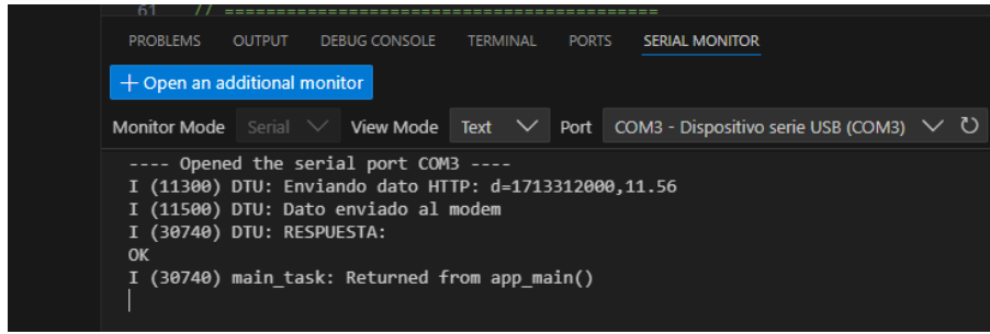
Figura 13: Prueba aislada del módem DTU. Se observa el envío de la trama d=timestamp,nivel y la respuesta OK recibida desde el servidor.
