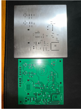
Figura 2: Stencil utilizado para la aplicación de pasta de soldar sobre los pads de la PCB.
