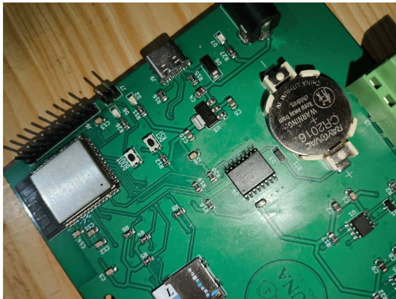
Figura 6: Circuito integrado DS3231 soldado en la PCB del proyecto como solución al problema del componente faltante.
