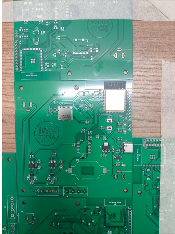
Figura 3: Colocación de los componentes sobre la PCB utilizando pinzas de precisión.
