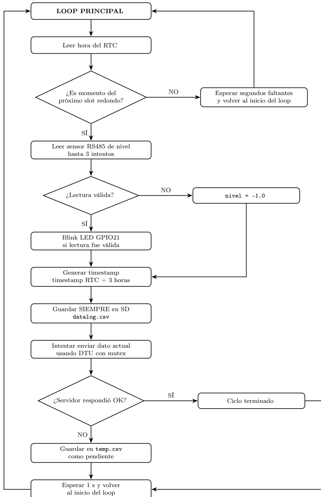
Figura 8: Secuencia lógica del loop principal de medición, almacenamiento y envío de datos.
