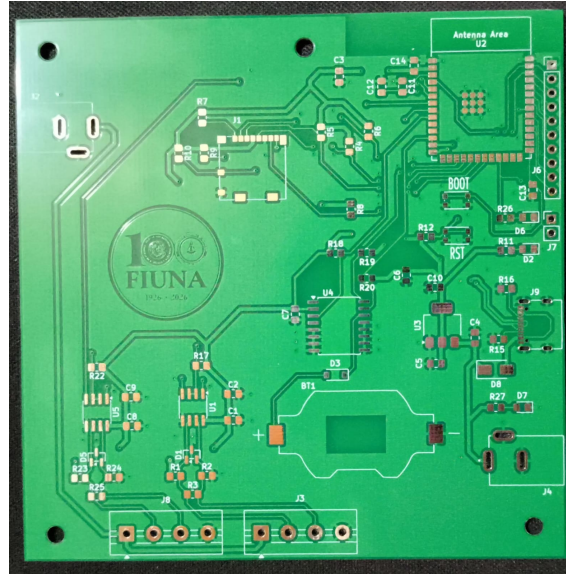
Figura 1: Revisión inicial de la PCB antes del montaje de los componentes.
