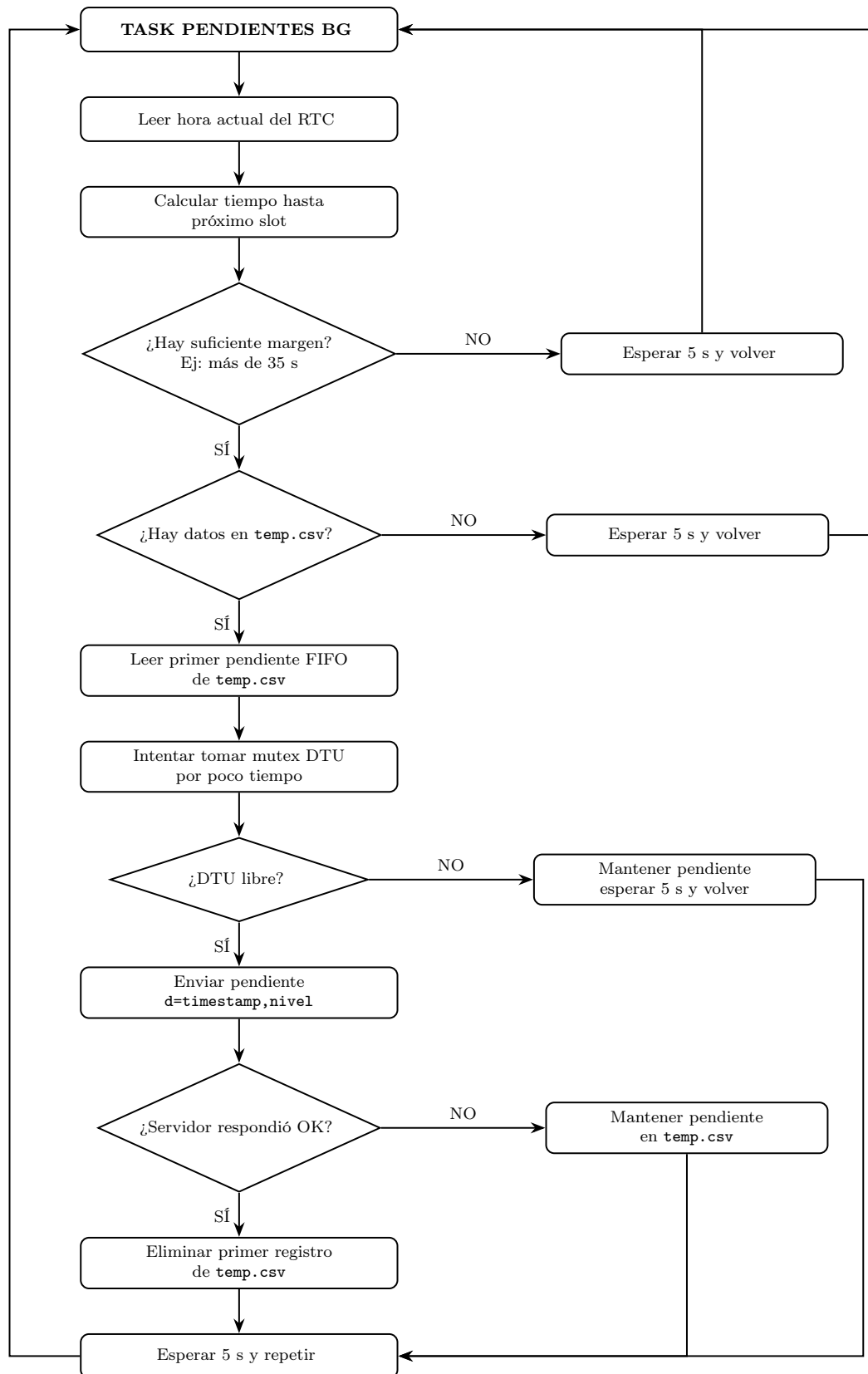
Figura 9: Flujo de la tarea en segundo plano para el reenvío de datos pendientes.
