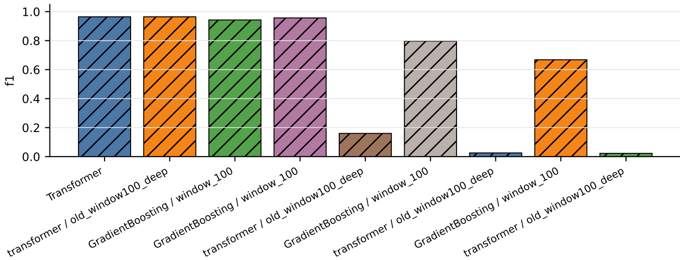
Conventional IDS F1
