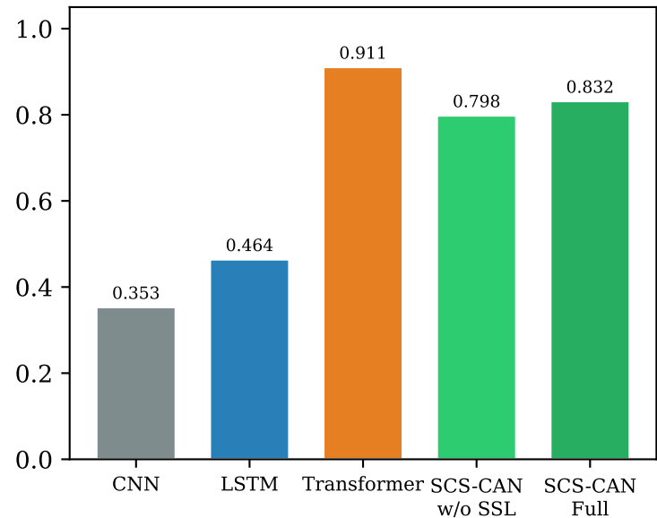
CrySyS
