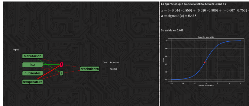
Figura 6.40: Etapa del forward pass en la que se ve en la ventana la función de activación dibujada junto con el punto que marca la salida de la función.
