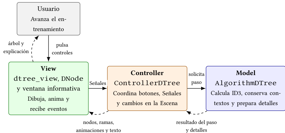
Figura 6.4: Separación de responsabilidades aplicada al árbol de decisión mediante el patrón Model-View-Controller.
