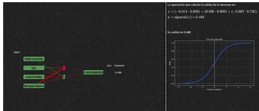
Figura 6.39: Etapa del forward pass en la que se ve en la ventana la función de activación dibujada junto con el punto que marca la salida de la función.
