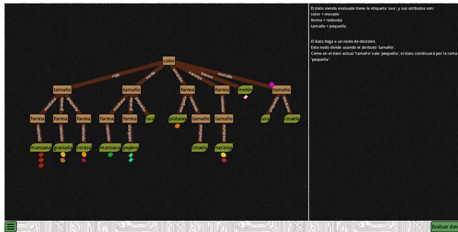
Figura 6.21: Árbol de decisión en medio del proceso de evaluación del dataset de frutas.
