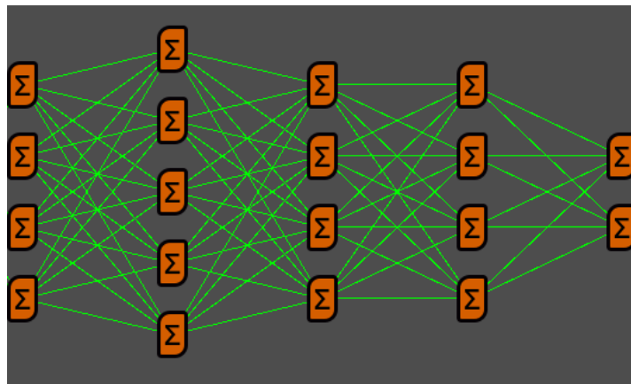
Figura 6.12: Primera arquitectura visual de la red neuronal, formada por capas, neuronas y conexiones densas entre capas consecutivas.
