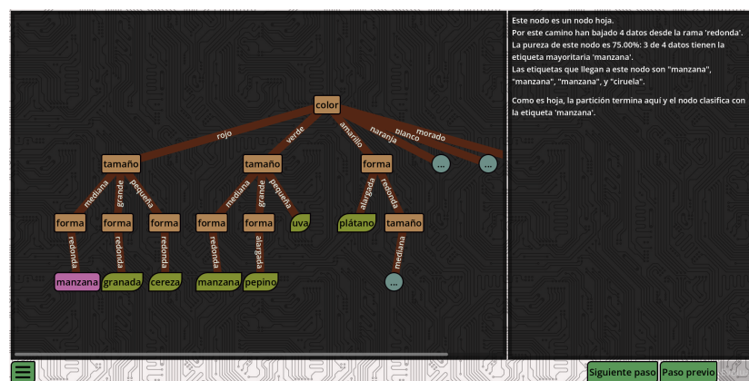
Figura 6.39: Ejemplo de un nodo resaltado durante el entrenamiento de un árbol de decisión.
