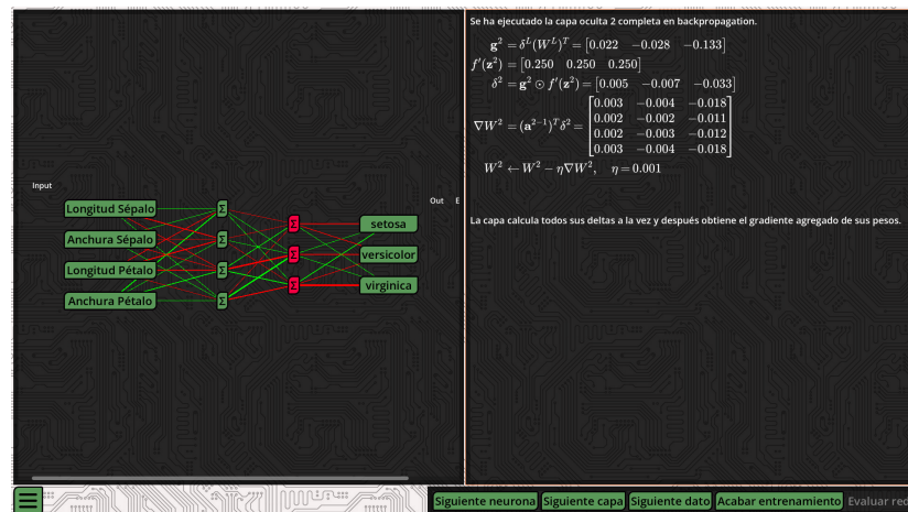
Figura 6.37: Texto y fórmulas de la retropropagación de la red por capas.
