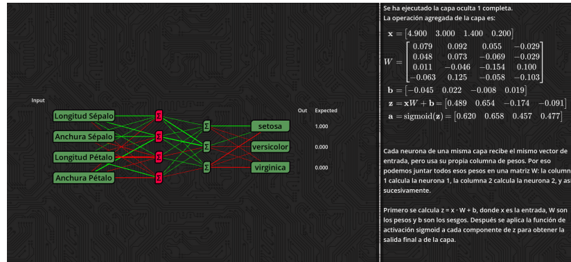
Figura 6.36: Texto y fórmulas de la propagación de la red por capas.
