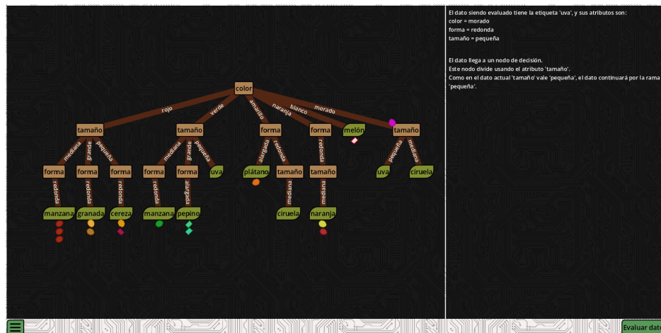
Figura 6.18: Árbol de decisión en medio del proceso de evaluación del dataset de frutas.
