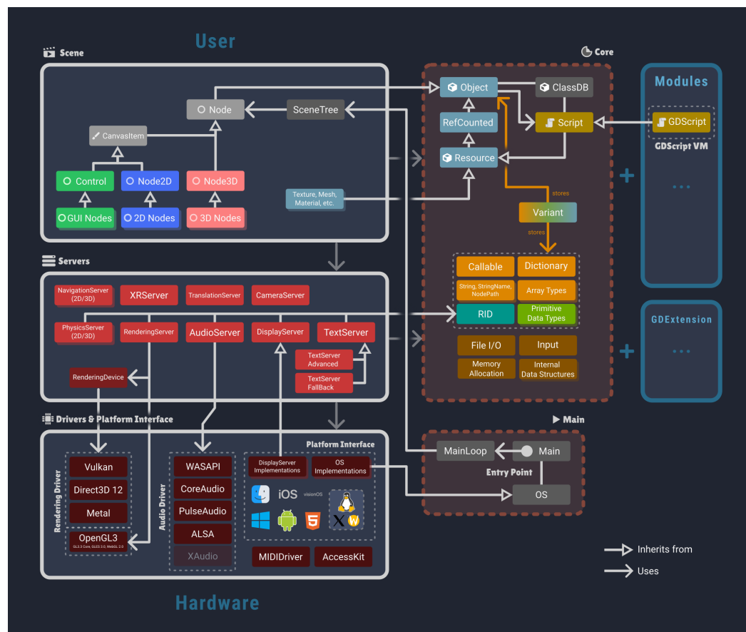
Figura 3.1: Diagrama general de la arquitectura de Godot.
