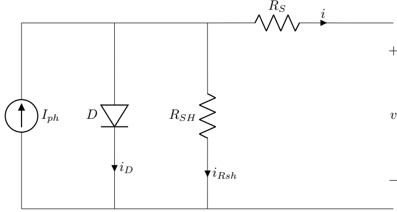
Figura 3.1: Modelo eléctrico equivalente de una celda solar con resistencia serie R_S y resistencia shunt R_{SH} .
