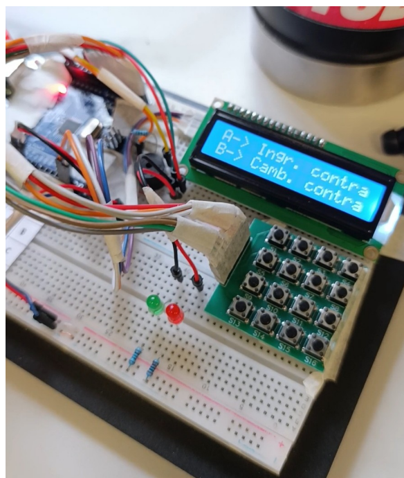
Figura 18. Montaje del circuito correspondiente al sistema de cerradura electrónica. Se observa la conexión del teclado matricial 4x4, la pantalla LCD 16x2 con interfaz I2C, los indicadores luminosos (LED rojo y verde), el buzzer de alarma y el microcontrolador ATmega328P. Fuente: elaboración propia.
