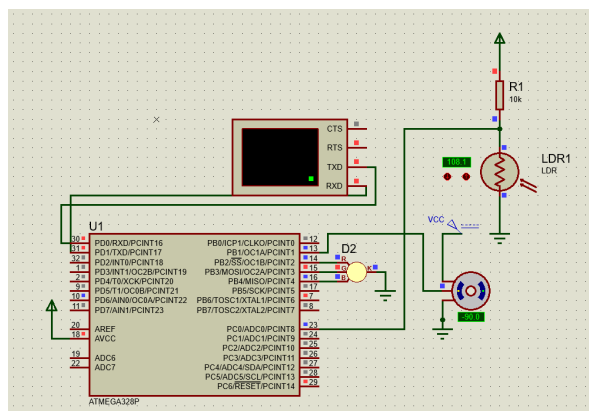
Figura 11. Simulación en Proteus del sistema de detección de color. Se observa la variación de la señal del LDR y la correspondiente respuesta del servomotor y de la tira LED. Fuente: elaboración propia.
