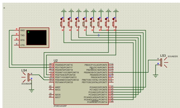
Figura 14. Simulación en Proteus del sistema de piano electrónico. Se observa la activación de los pulsadores, la generación de tonos en el buzzer y la respuesta del microcontrolador ATmega328P configurado con interrupciones PCINT . Fuente: elaboración propia.
